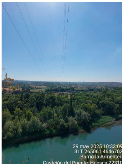
Línea cruzando río Cinca con salvapájaros
