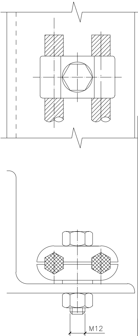
DETALLE 2 SIN ESCALA
