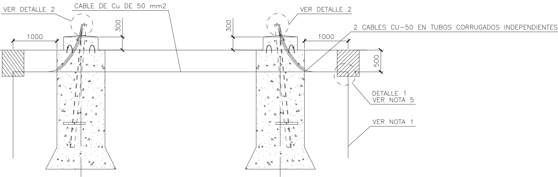
ALZADO
