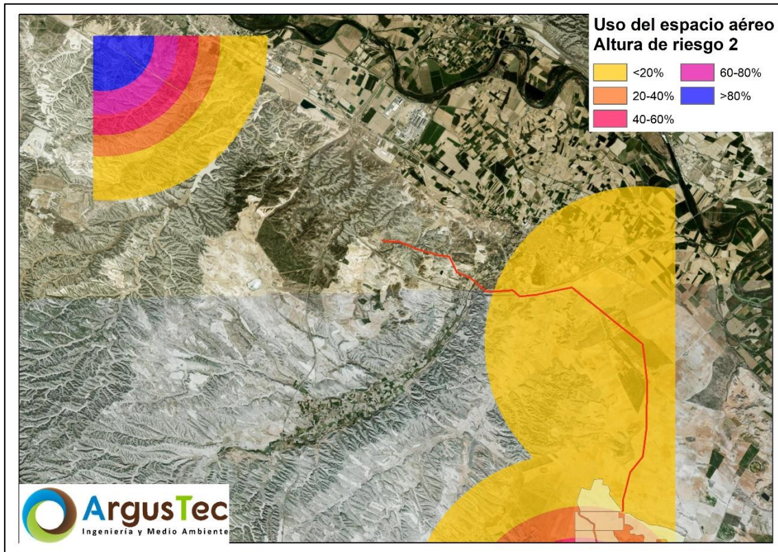
Figura 3 Análisis Kernel del uso e intensidad del espacio aéreo por las aves observadas en el entorno de la zona de estudio desde los puntos de observación de LAAT Fuentes.
