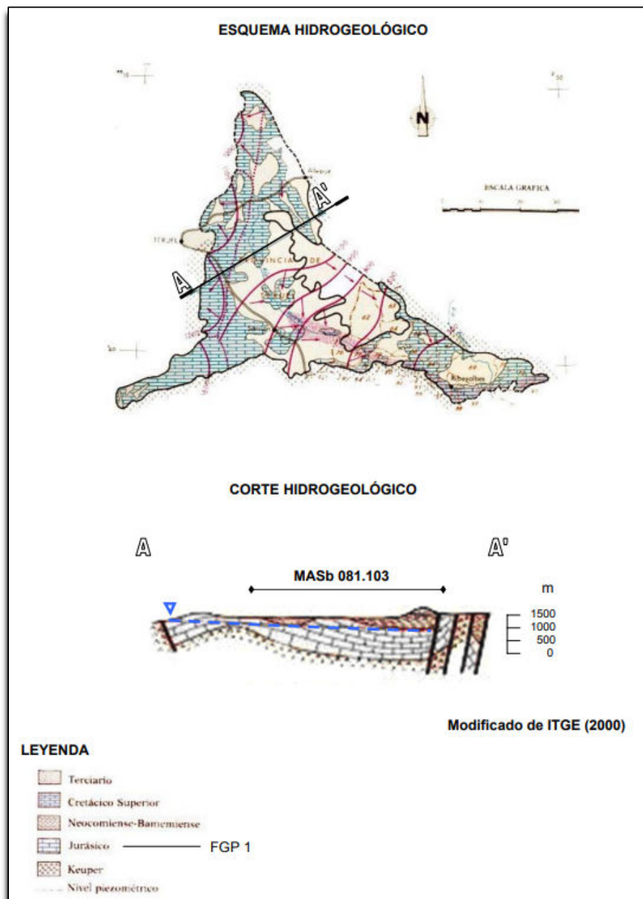
Figura nº 16. Corte y esquema hidrogeológico de la MASb 081.103 Javalambre Oriental.
