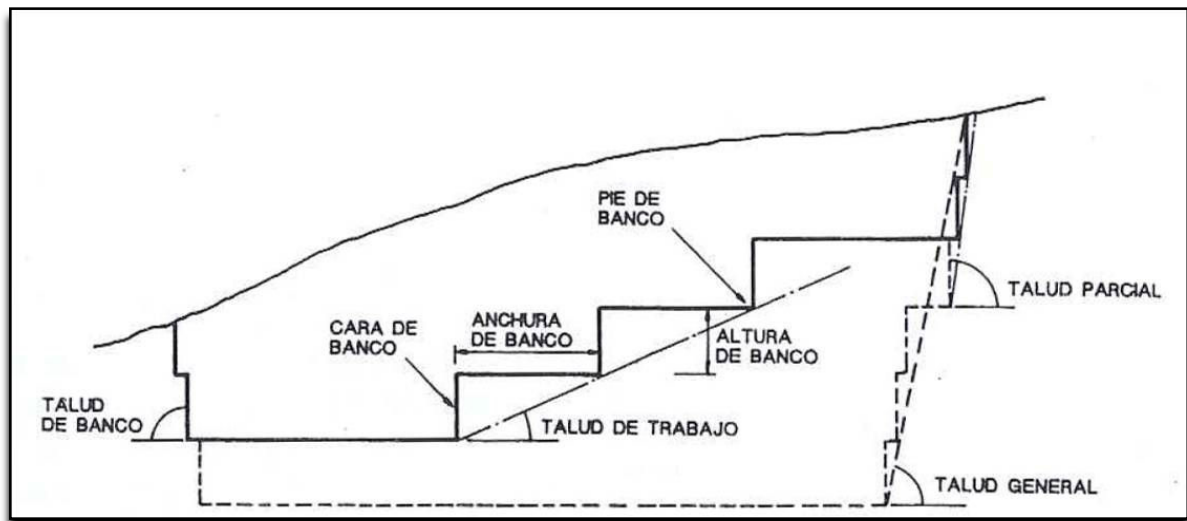
Figura nº 37. Terminología empleada en una explotación a cielo abierto. LÓPEZ JIMENO 1995.
