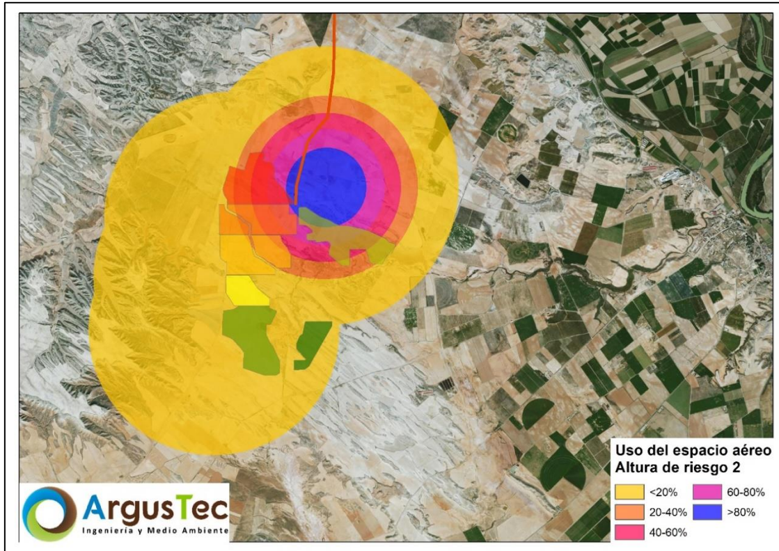
Figura 3 Análisis Kernel del uso e intensidad del espacio aéreo por las aves observadas en el entorno de la zona de estudio desde los puntos de observación Valdompere 3
