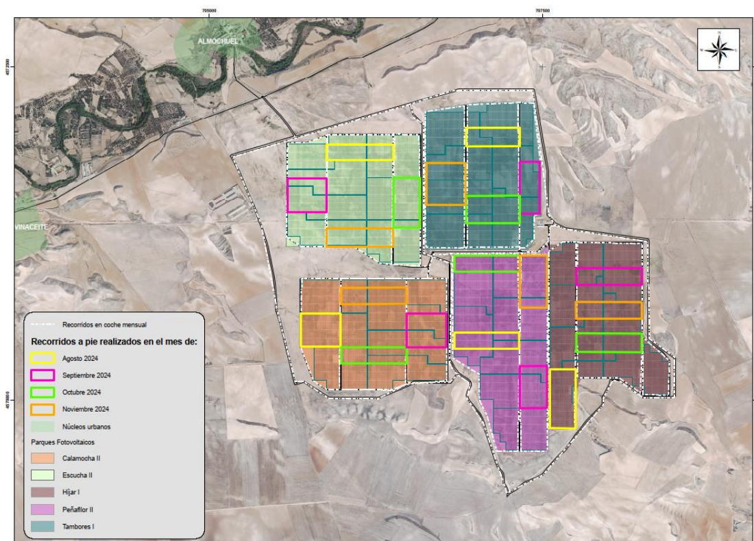
Figura 7. Recorridos de seguimiento de siniestralidad de avifauna dentro y en los alrededores de las 5 plantas fotovoltaicas
