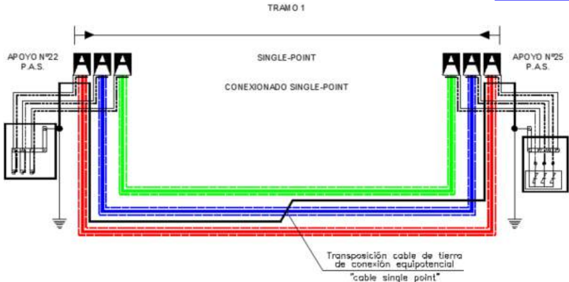
Esquema de conexionado "Single Point"
