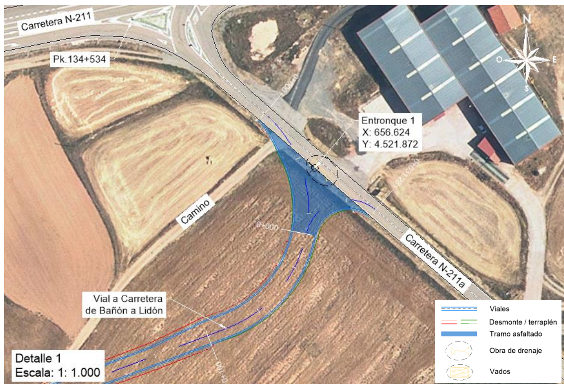
Entronque 1 con Carretera N-211a
