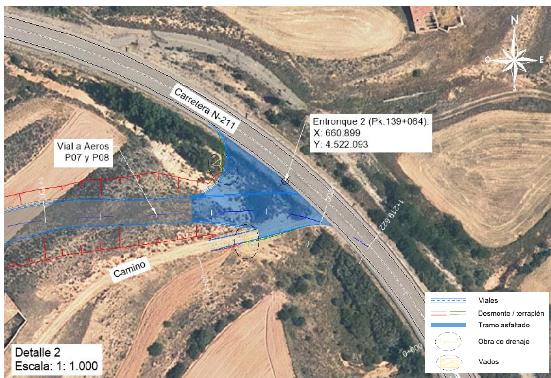
Entronque 2 con Carretera N-211
