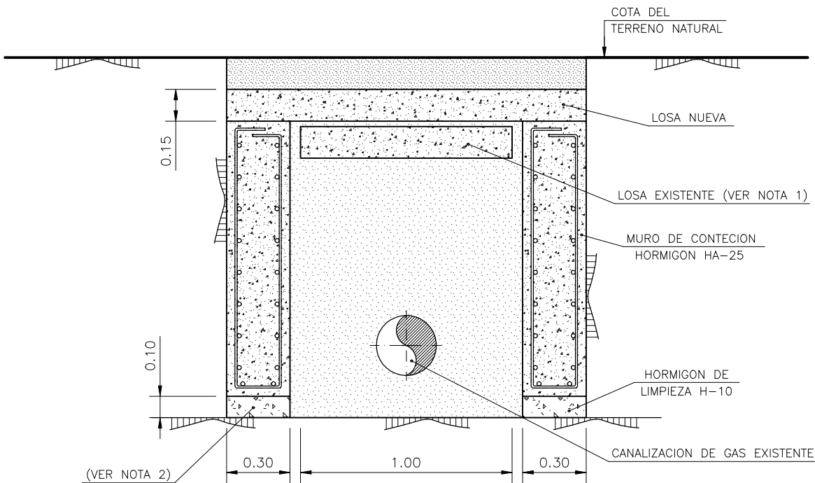
SECCION
