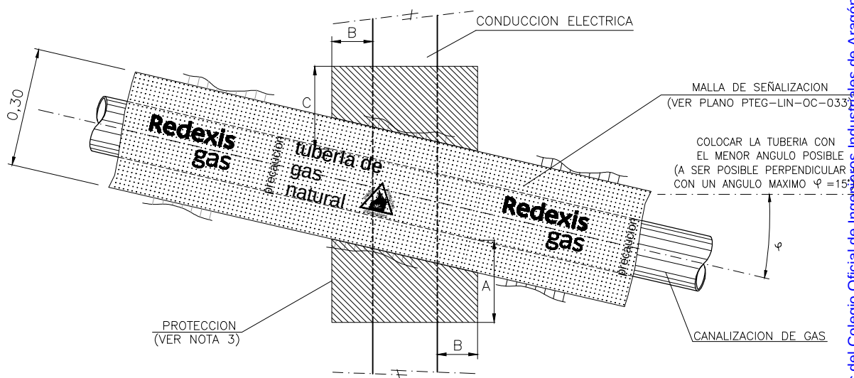
DIMENSIONES PROTECCION
