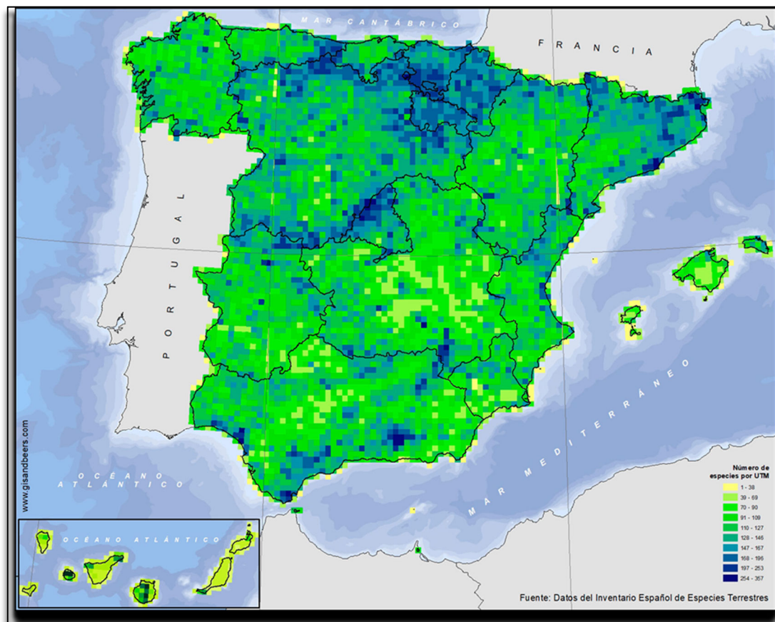
Figura nº 11. Mapas de “Riqueza de especies” en cuadrículas 10x10 km para la Península Ibérica. Fuente: Inventario del Patrimonio Natural y la Biodiversidad MITECO.
