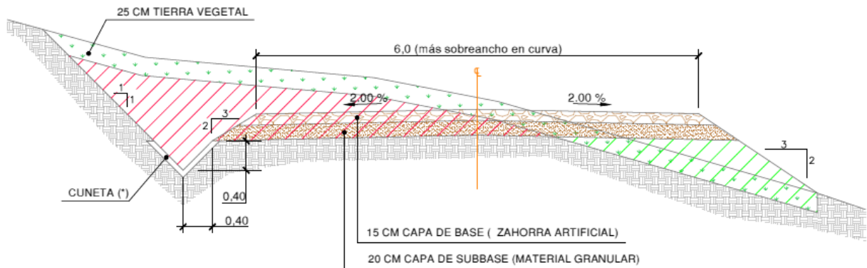
Imagen 8.Sección Vial Granular.
