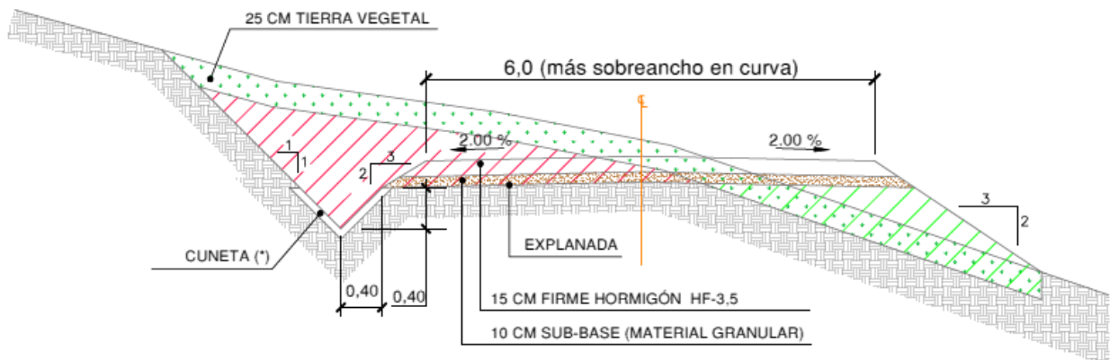
Imagen 9. Sección Vial Hormigonado.
