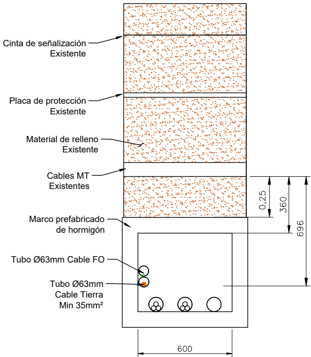
TIPO BT 2 TERNA HORMIGONADA EN CRUCE CON OTRAS LÍNEAS DE MEDIA TENSIÓN
