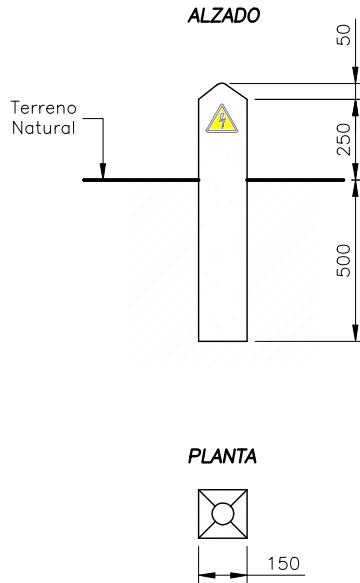
HITOS DE SEÑALIZACIÓN
