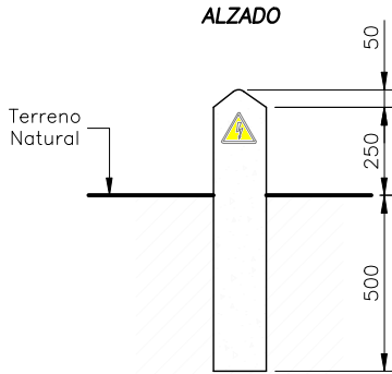
HITOS DE SEÑALIZACIÓN
