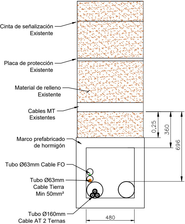
TIPO MT 1 TERNA HORMIGONADA EN CRUCE CON OTRAS LÍNEAS DE MEDIA TENSIÓN
