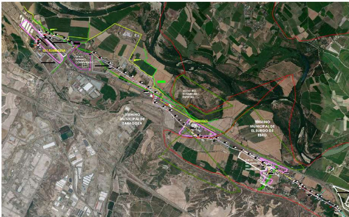
Situación de línea aero subterránea en TT.MM de Zaragoza y El Burgo de Ebro, desde SET Alumalsa, realizando entrada-salida en SET Prydes hasta entronque con línea existente Prydes-El Burgo en apoyo 99 existente.
