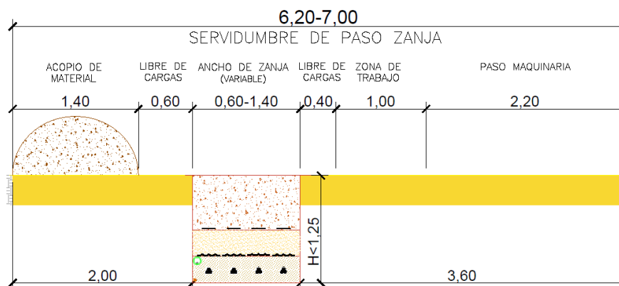
Ilustración 1: Sección transversal de detalle de servidumbre de zanja
