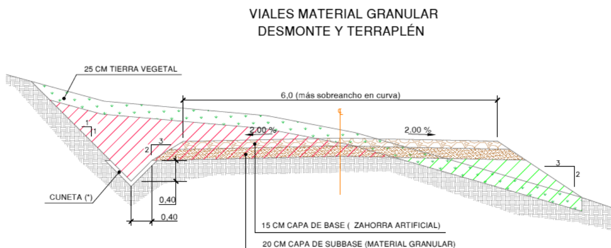
Imagen 8. Sección Vial Granular.
