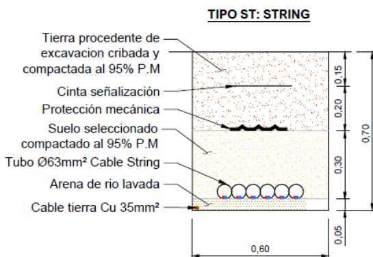
Ilustración 6: Detalle de la zanja tipo string de BT
