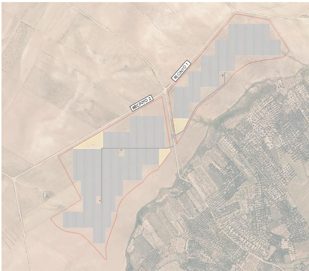
Ilustración 5: Disposición de viales
