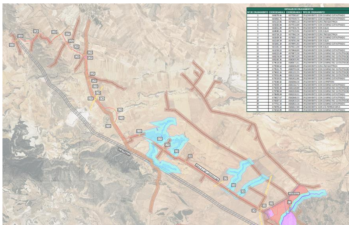
Ilustración 11: Afecciones del módulo de generación fotovoltaico y la línea de evacuación
