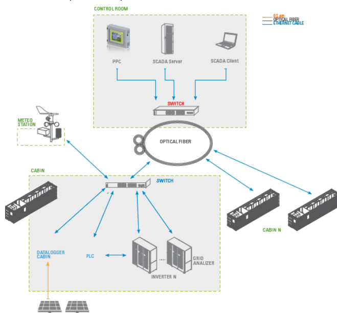
Ilustración 10: Esquema del sistema de monitorización del módulo
