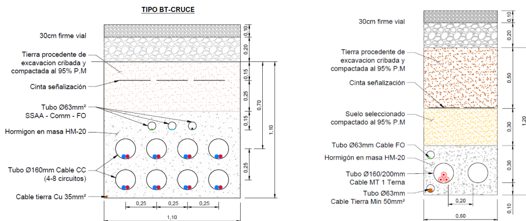
Ilustración 7: Detalles de las zanjas tipo cruce para BT (izda.) y MT (dcha.)
