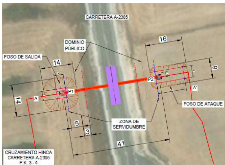
Ilustración 9: Detalle cruce línea de evacuación subterránea con carretera A-2305
