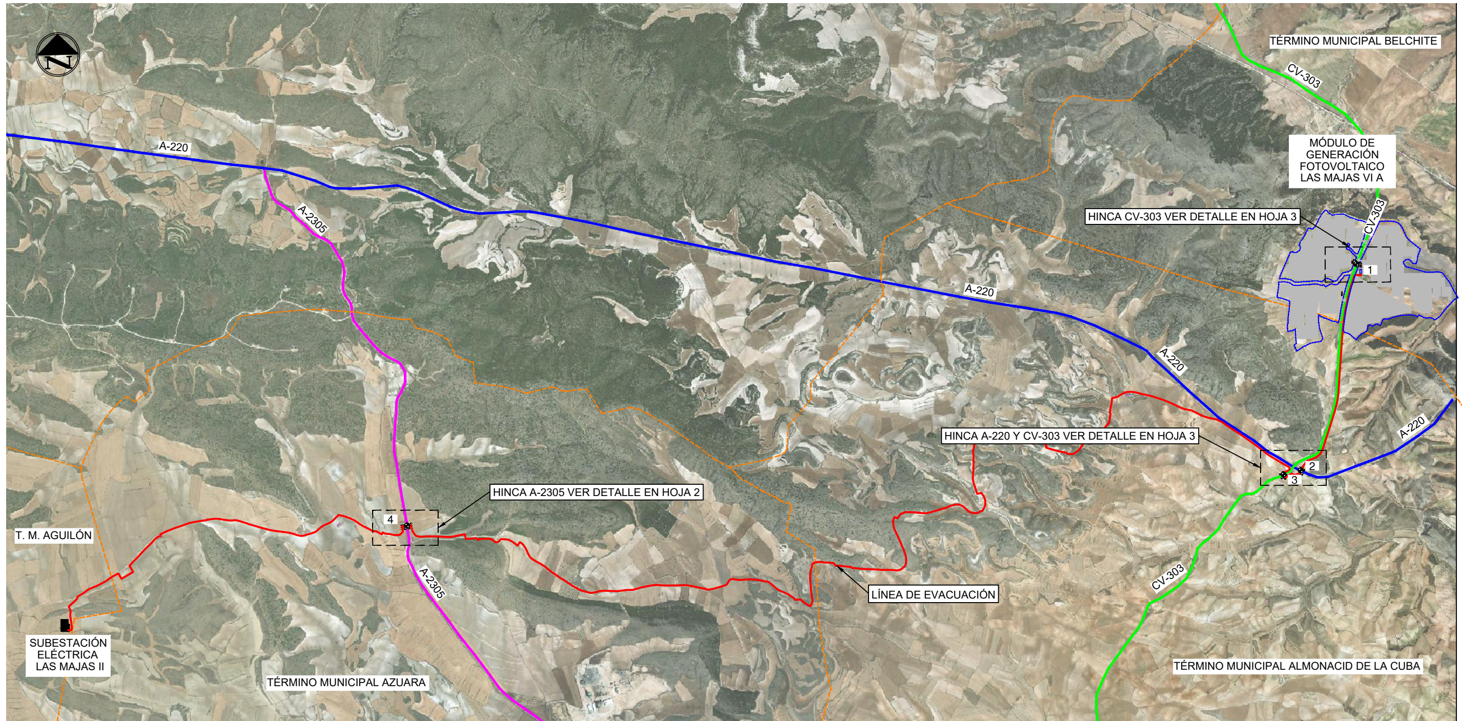
1 PLANTA GENERAL Y LÍNEA DE EVACUACIÓN Escala: 1:30.000
