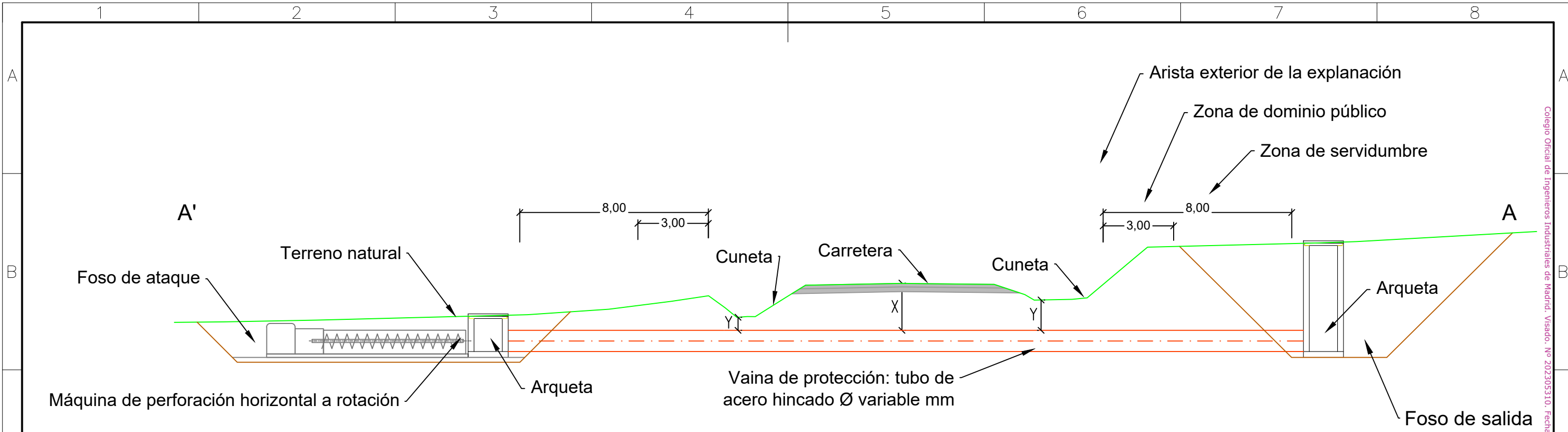
1 SECCIÓN HINCA CARRETERA Escala: 6/1
