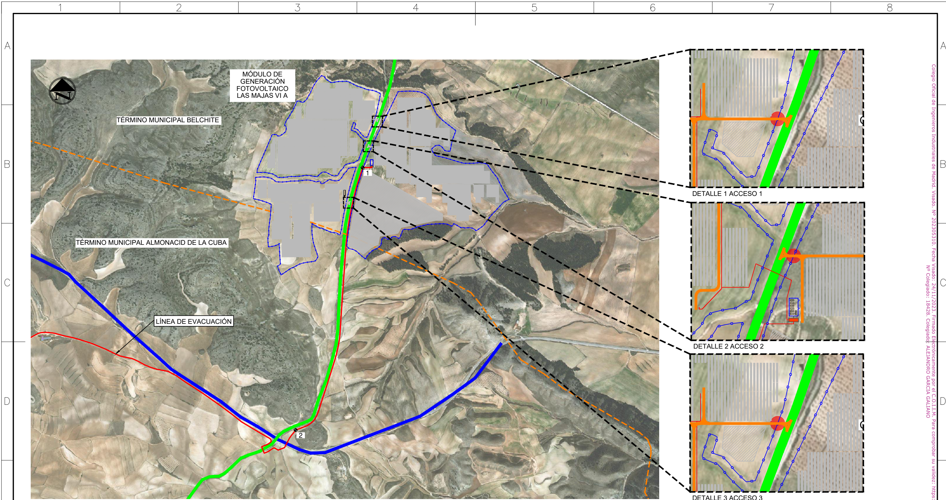
1 PLANTA GENERAL Y LÍNEA DE EVACUACIÓN Escala: 1:30.000
