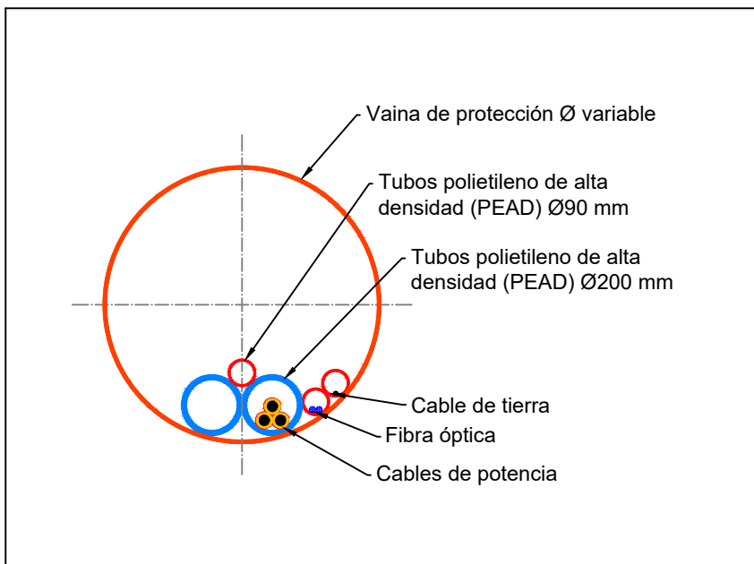
2 DETALLE SECCIÓN B-B' Escala: 8/1
