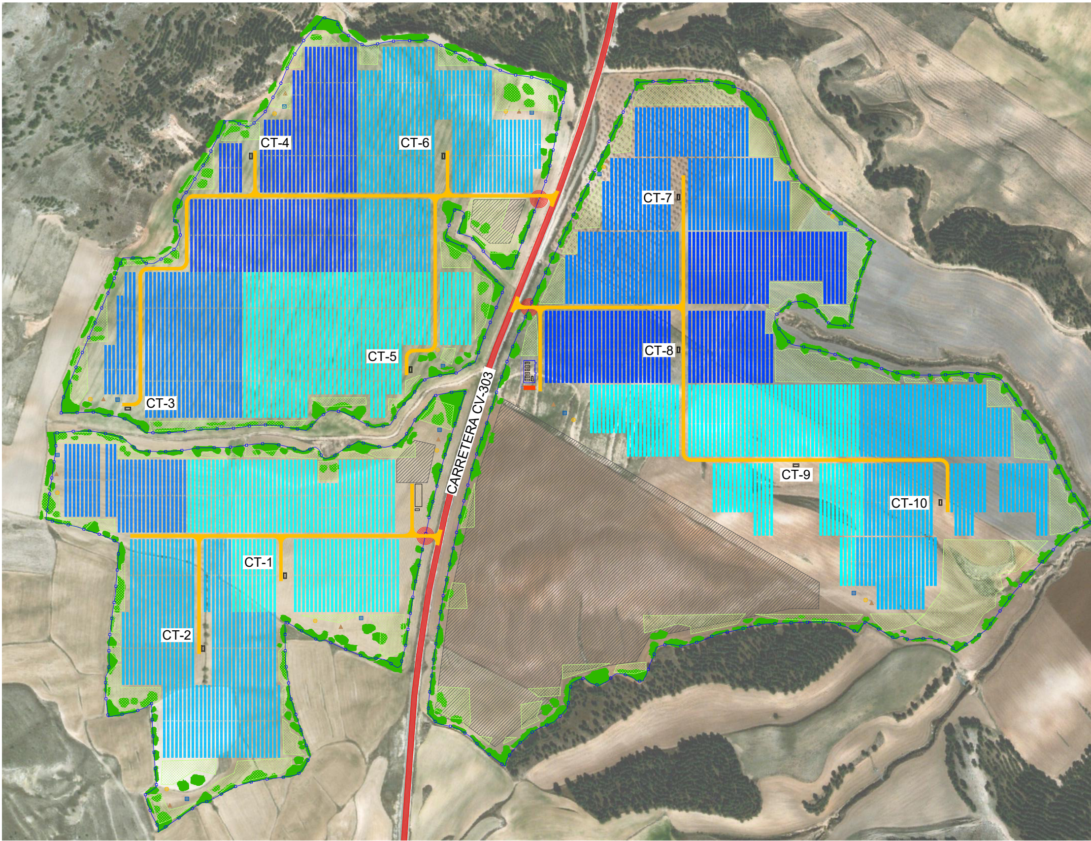
1 PLANTA GENERAL Escala: 1:5.000
