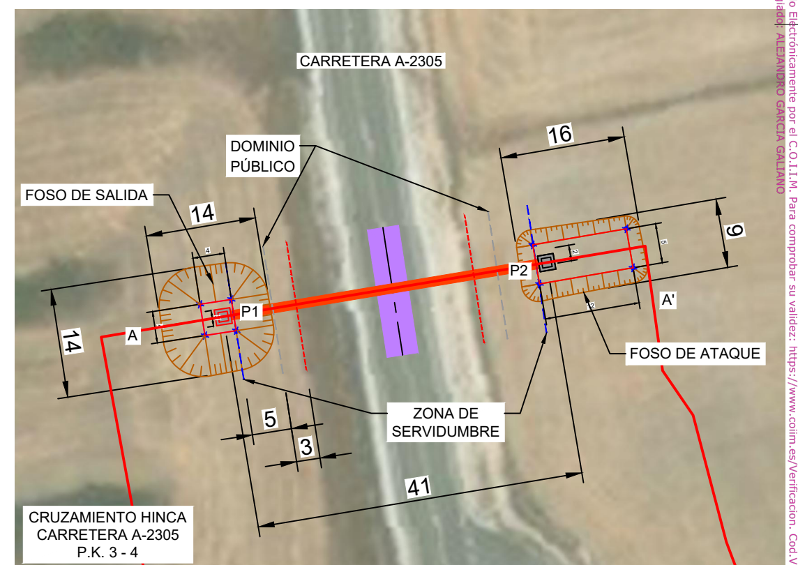
3 SECCIÓN HINCA CARRETERA A-2305 Escala: 1.5/1
