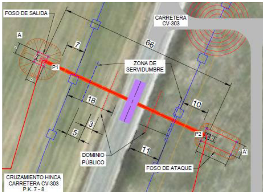
Ilustración 6: Detalle cruzamiento zanja de media tensión con carretera CV-303
