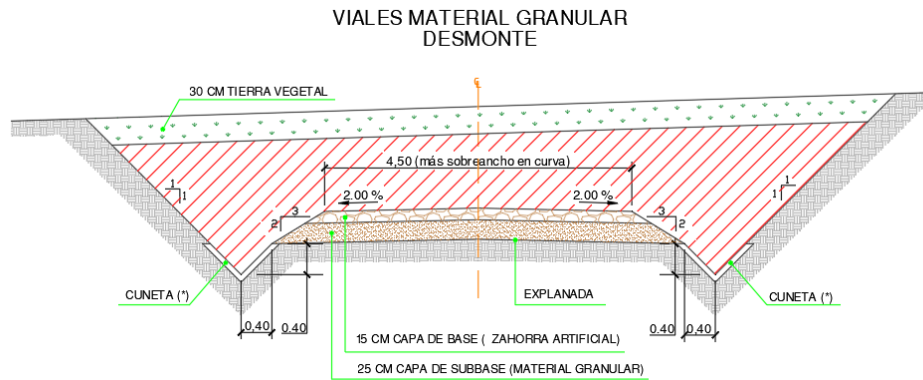
Ilustración 14 Sección tipo viales para pendientes < 10%. Vial primario.
