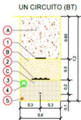
Ilustración 9 Especificación de la zanja de la torre de medición.
