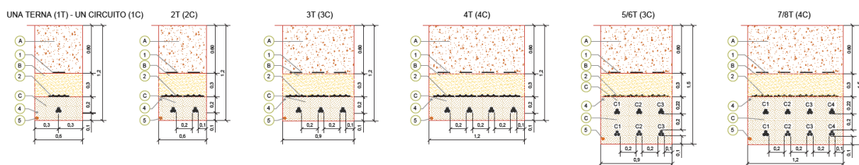
Ilustración 22 Zanjas para circuitos directamente enterrados.
