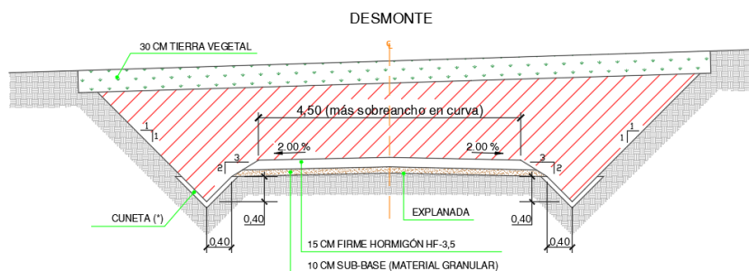
Ilustración 15 Sección tipo viales para pendientes >14%.
