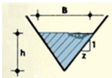
Ilustración 18 Cuneta tipo
