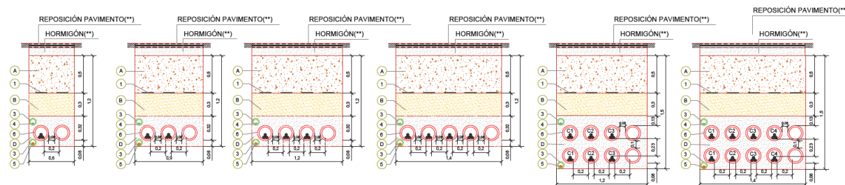
Ilustración 25 Zanjas para circuitos directamente enterrados bajo calzada.
