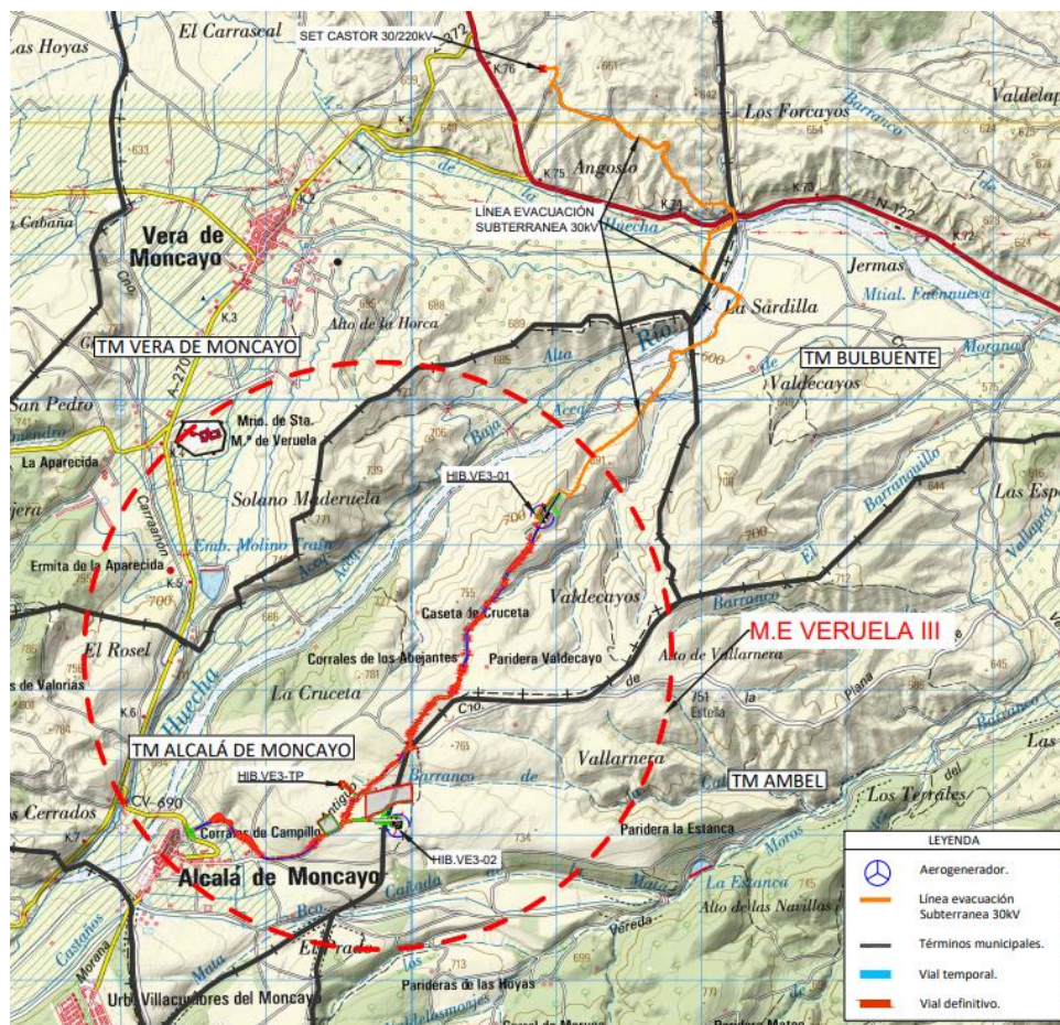
Ilustración 6 Emplazamiento general del Módulo Eólico Veruela III
