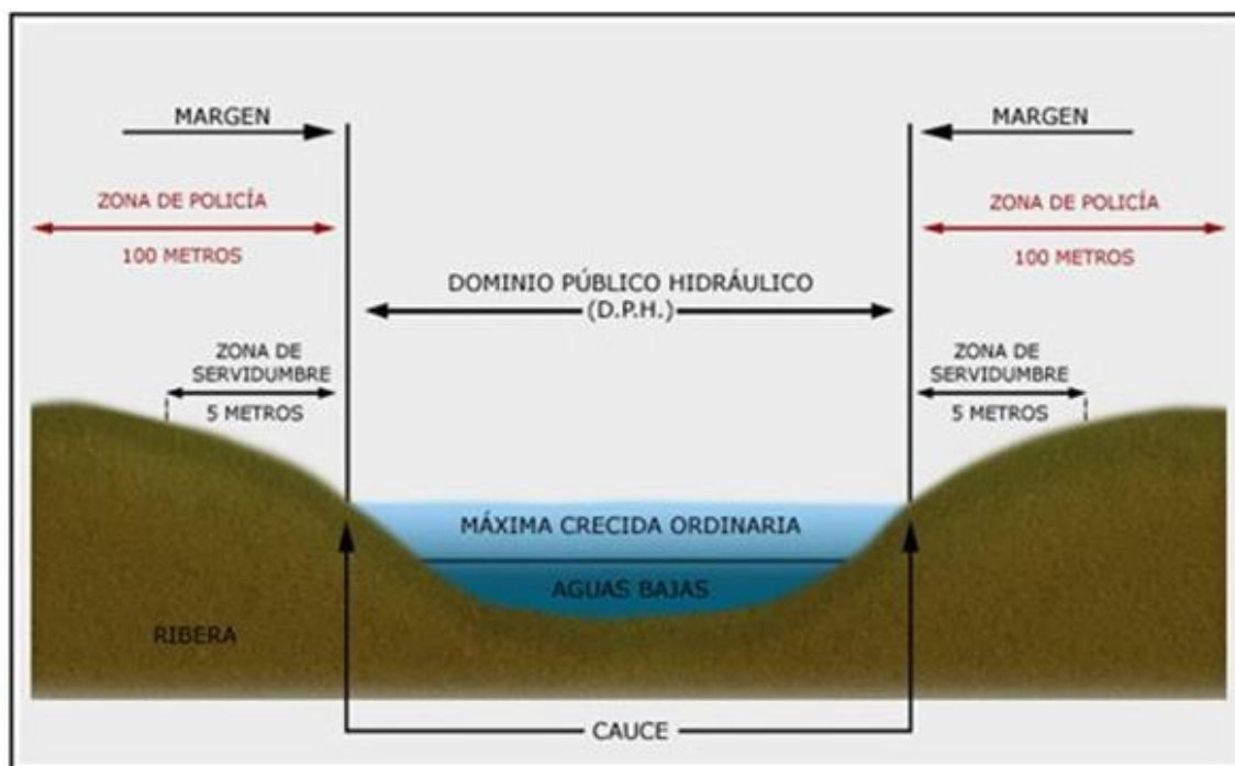
Ilustración 3 Distancias mínimas a construcciones
