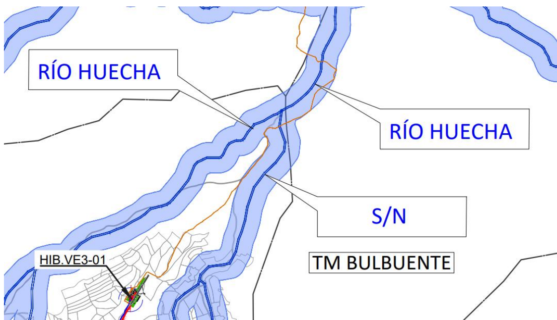
Ilustración 4 Cruce con río Huecha
