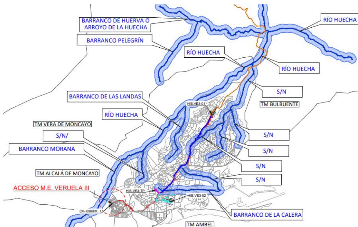
Ilustración 2 Módulo Eólico Veruela III y afecciones a la confederación hidrográfica del Duero
