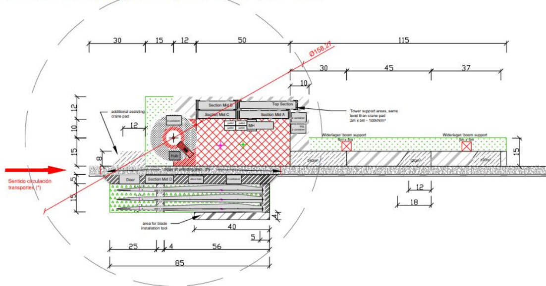
Ilustración 19 Plataforma utilizada / HIBVE3-01
