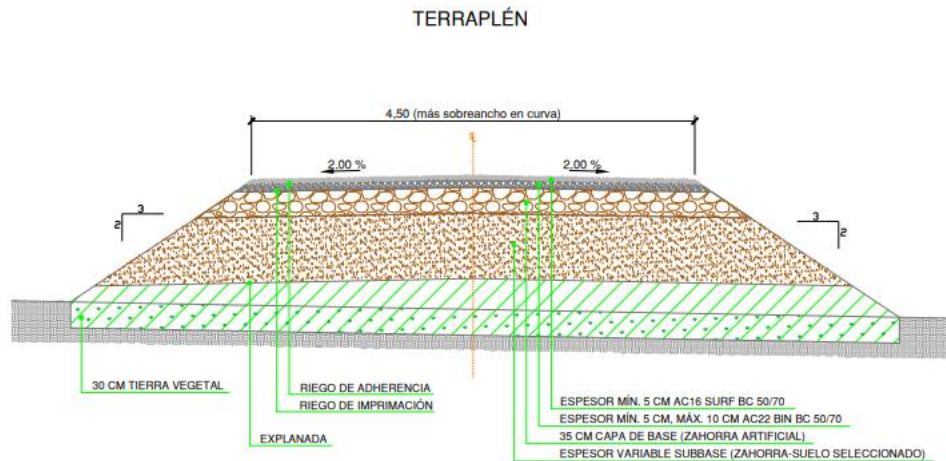
Ilustración 13 Sección tipo viales para pendientes < 10%. Vial Aglomerado
