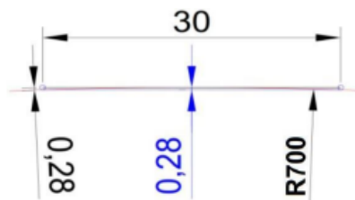
Ilustración 16 Tolerancia irregularidades del suelo.
