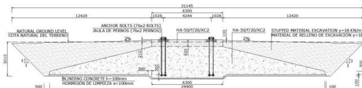
Ilustración 21 Sección de la cimentación: dimensiones establecidas.
