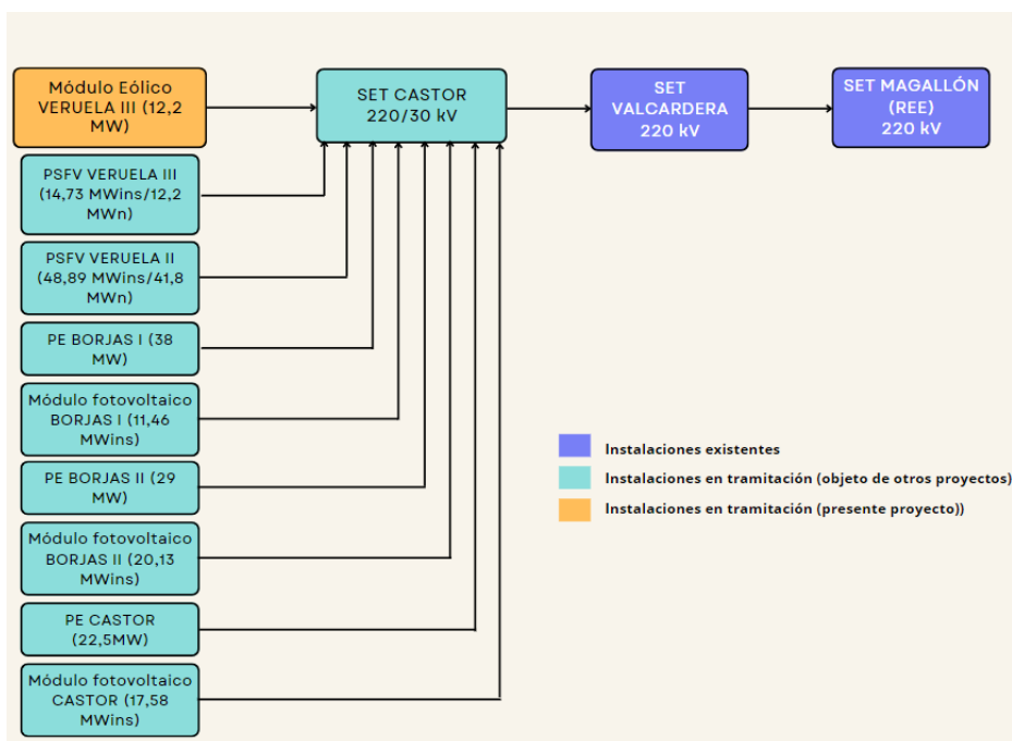
Ilustración 12 Conexión SET Castor
