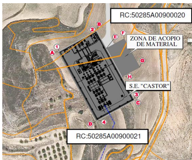
Ilustración 11 Infraestructura de Evacuación - SET Castor
