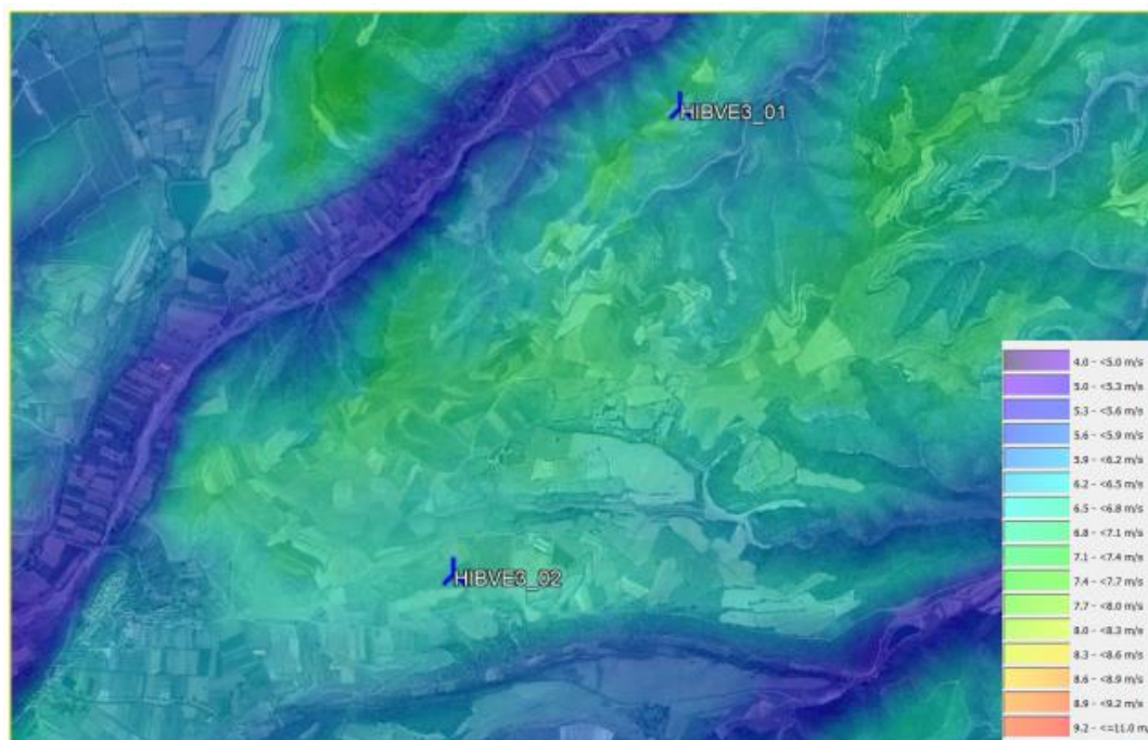
Ilustración 8 Mapa de recurso eólico a 120,9 m de altura.
