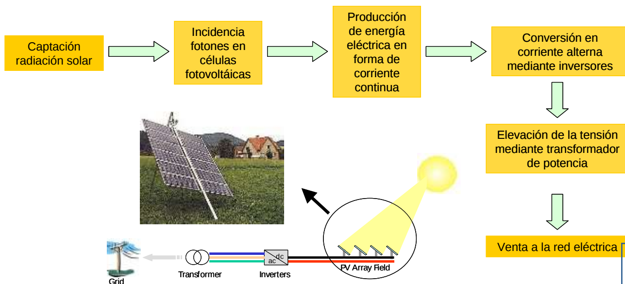
Figura 7: Principio de Funcionamiento Instalación FV.
