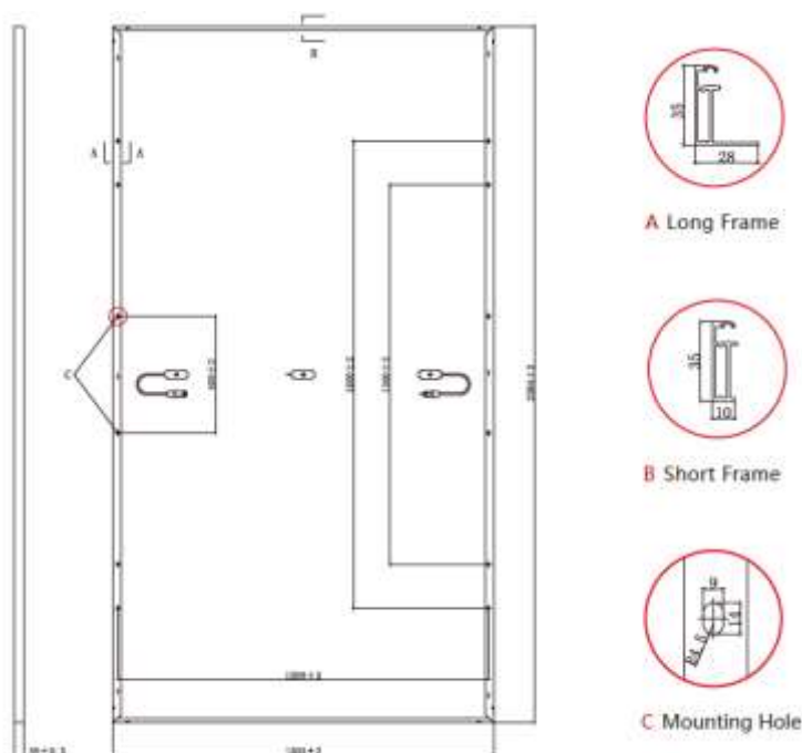
Figura 9: Dimensiones del Módulo.
