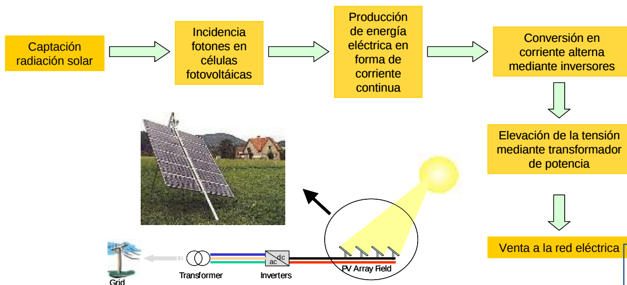
Figura 8: Principio de Funcionamiento Instalación FV.
