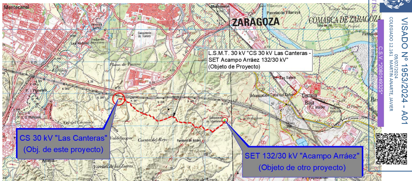
A continuación, se muestra el plano de localización de la L.S.M.T.:
