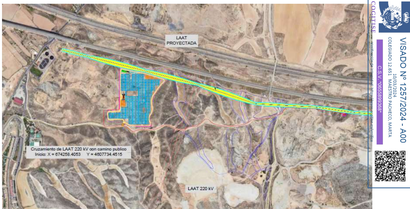
Figura 10: Líneas eléctricas.
