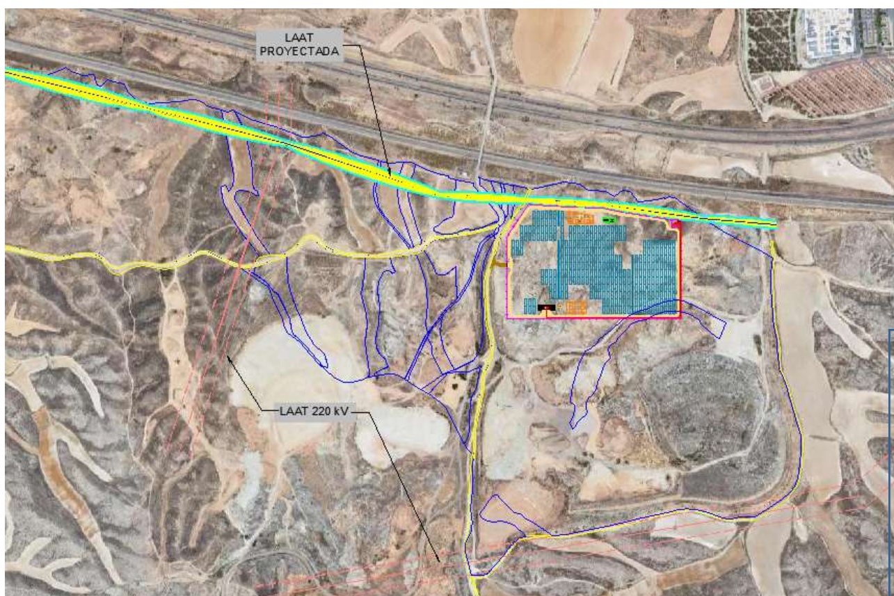
Figura 20: Líneas eléctricas.
