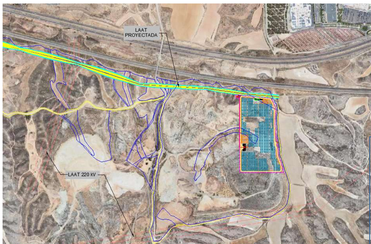
Figura 20: Líneas eléctricas.
