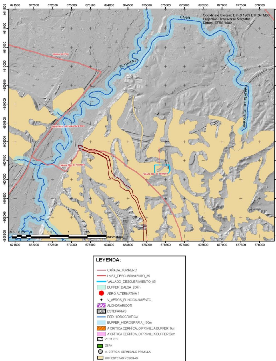
Figura 4.- Alternativa 2 de ubicación de la PSFV EL DESCUBRIMIENTO 85 y la línea soterrada de evacuación.
