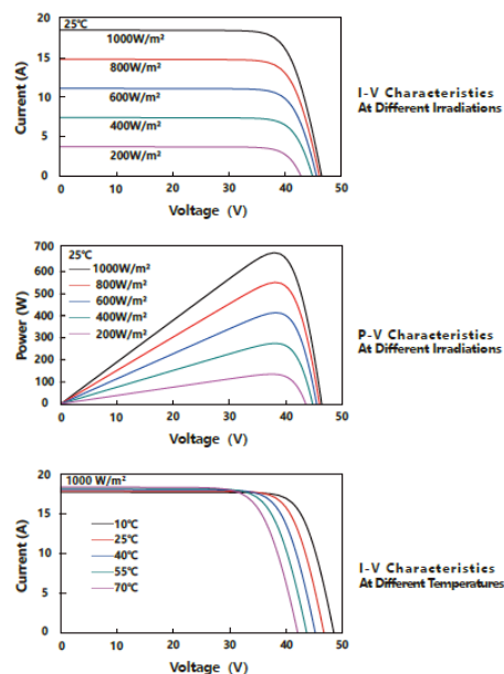
Figura 32.- Curvas Características JW-HD132N.
