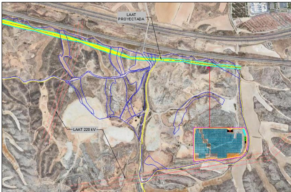
Figura 91.- Líneas eléctricas.
