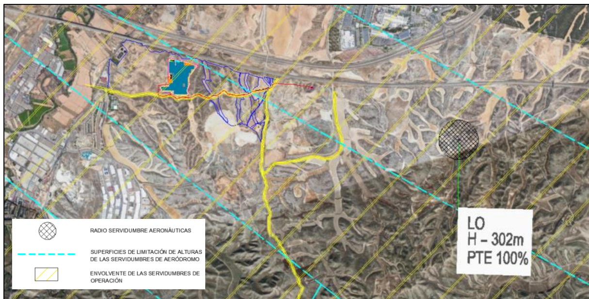
Figura 97.- Servidumbres aeronáuticas.
