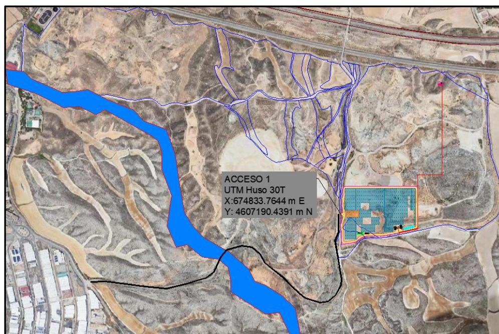
Figura 8.- Acceso al Parque Solar FV (en color negro).
