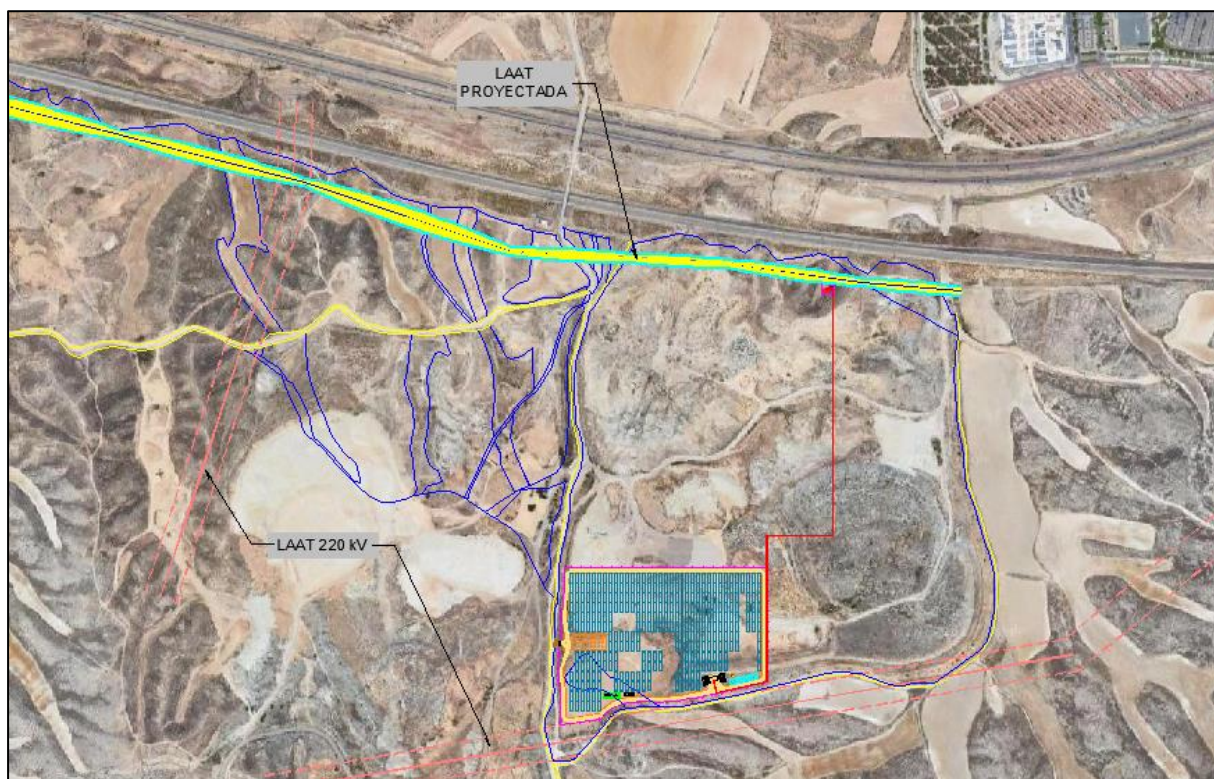
Figura 22.- Líneas eléctricas.
