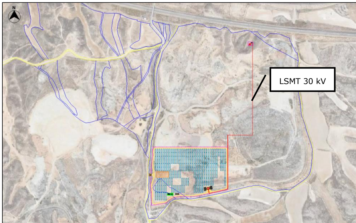
Figura 33.- Localización LSMT.
