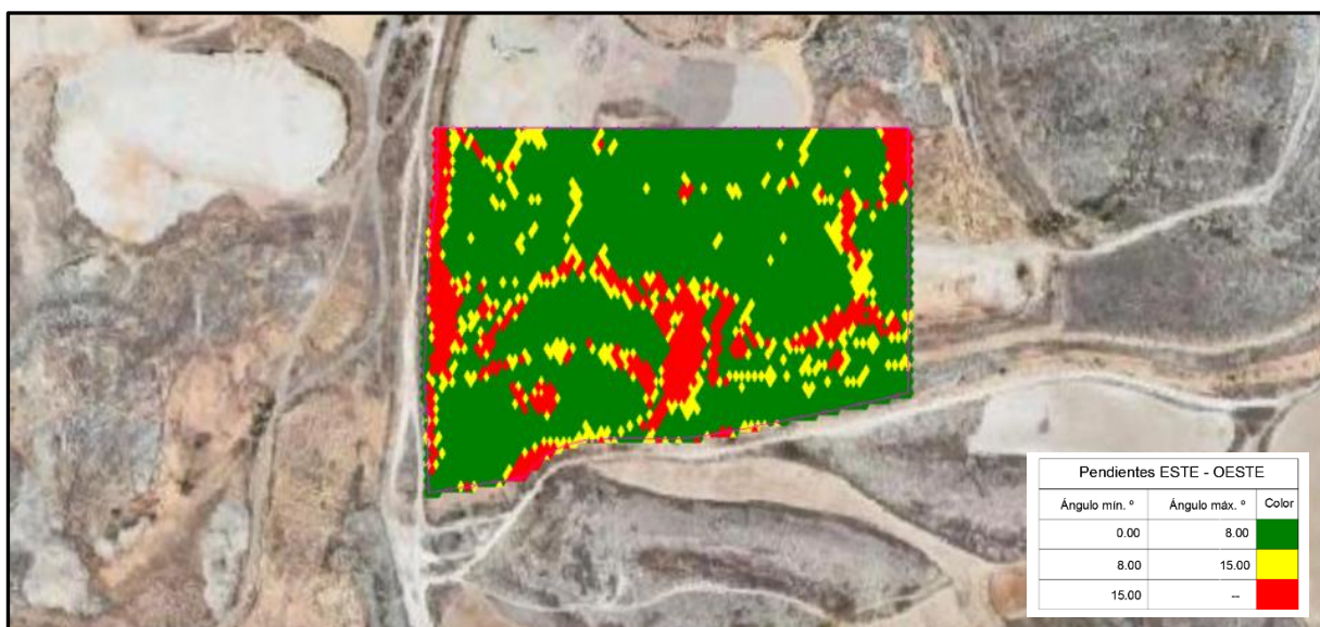
Figura 11.- Pendientes E-O.
