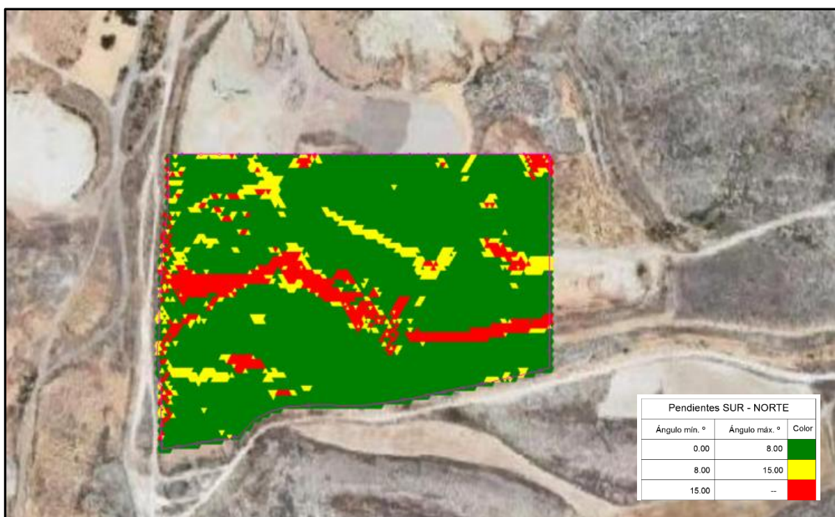
Figura 9.- Pendientes S-N.
