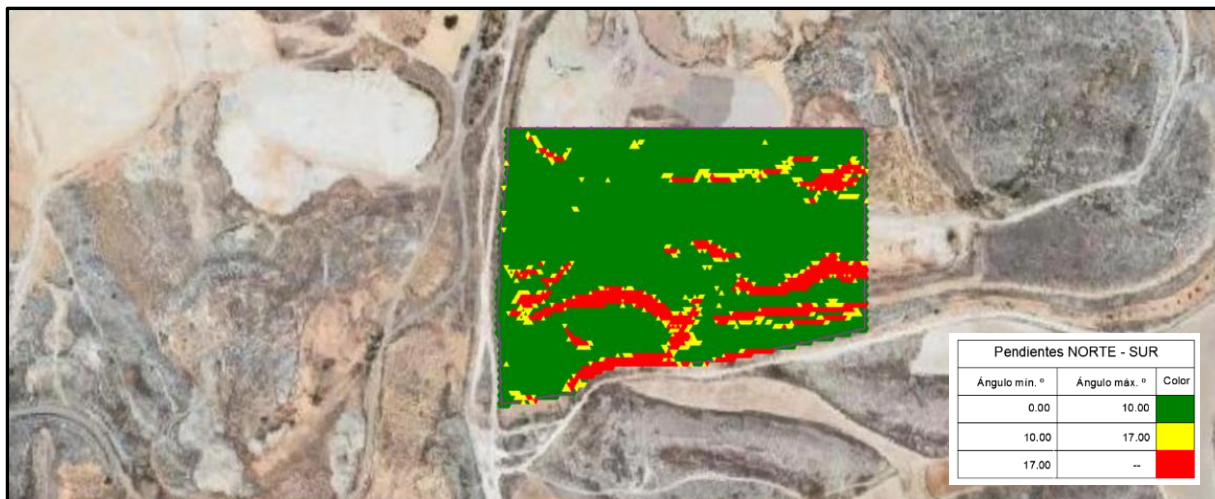
Figura 10.- Pendientes N-S.
