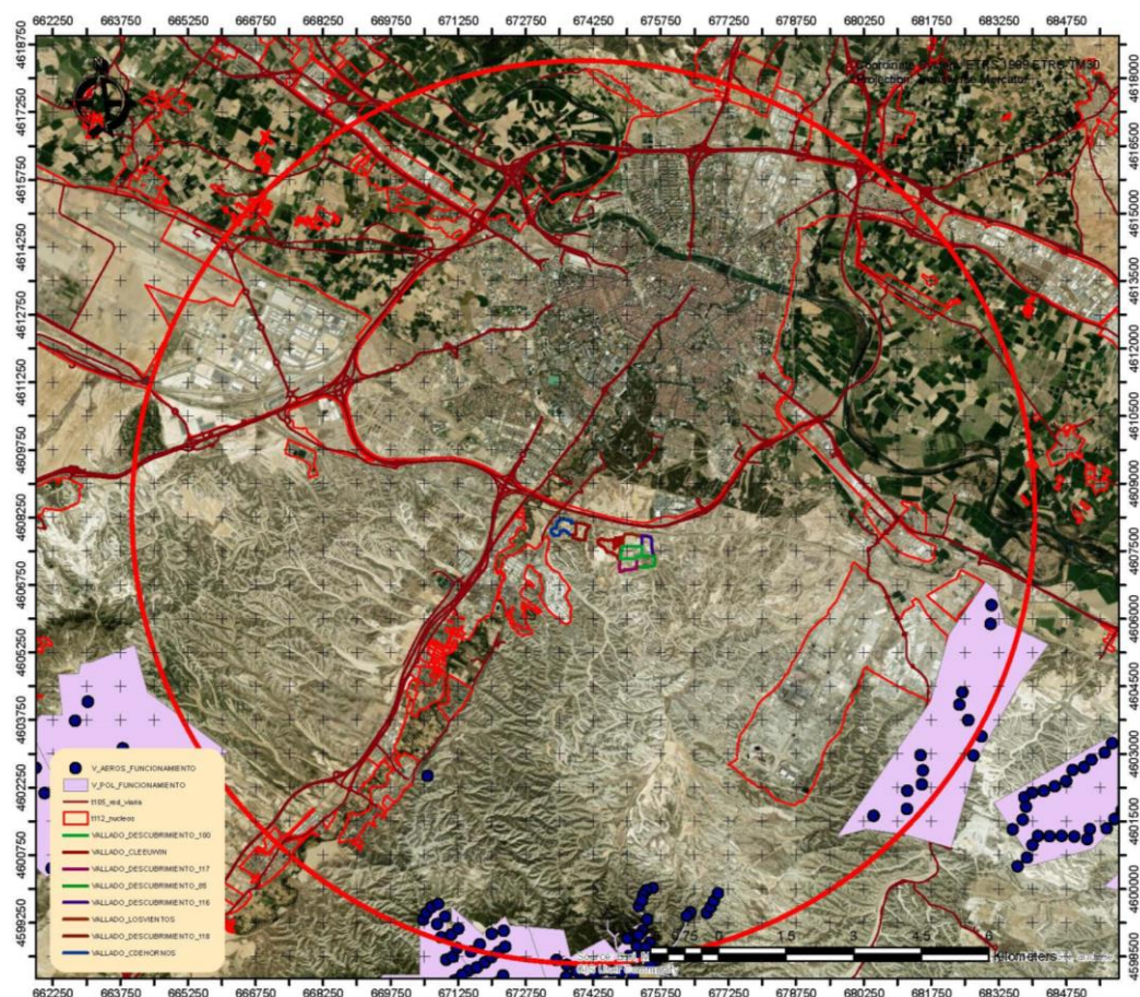
Figura 27.- Parques Eólicos.
