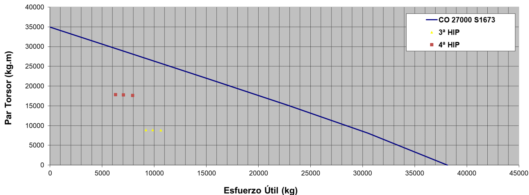
ESFUERZO ÚTIL vs TORSIÓN - (C.S.=1,20)
