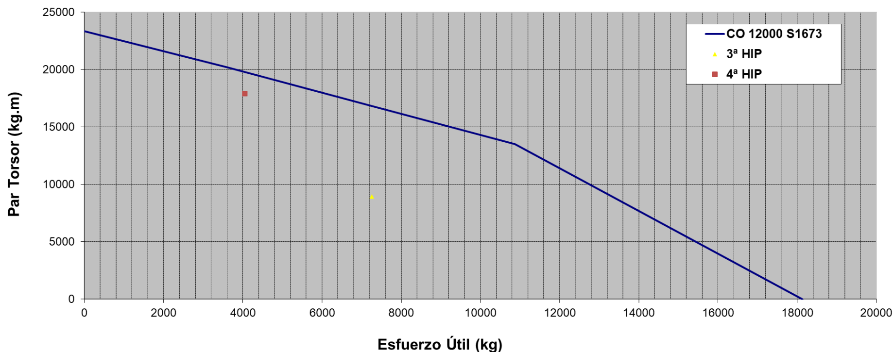
ESFUERZO ÚTIL vs TORSIÓN - (C.S.=1,20)
