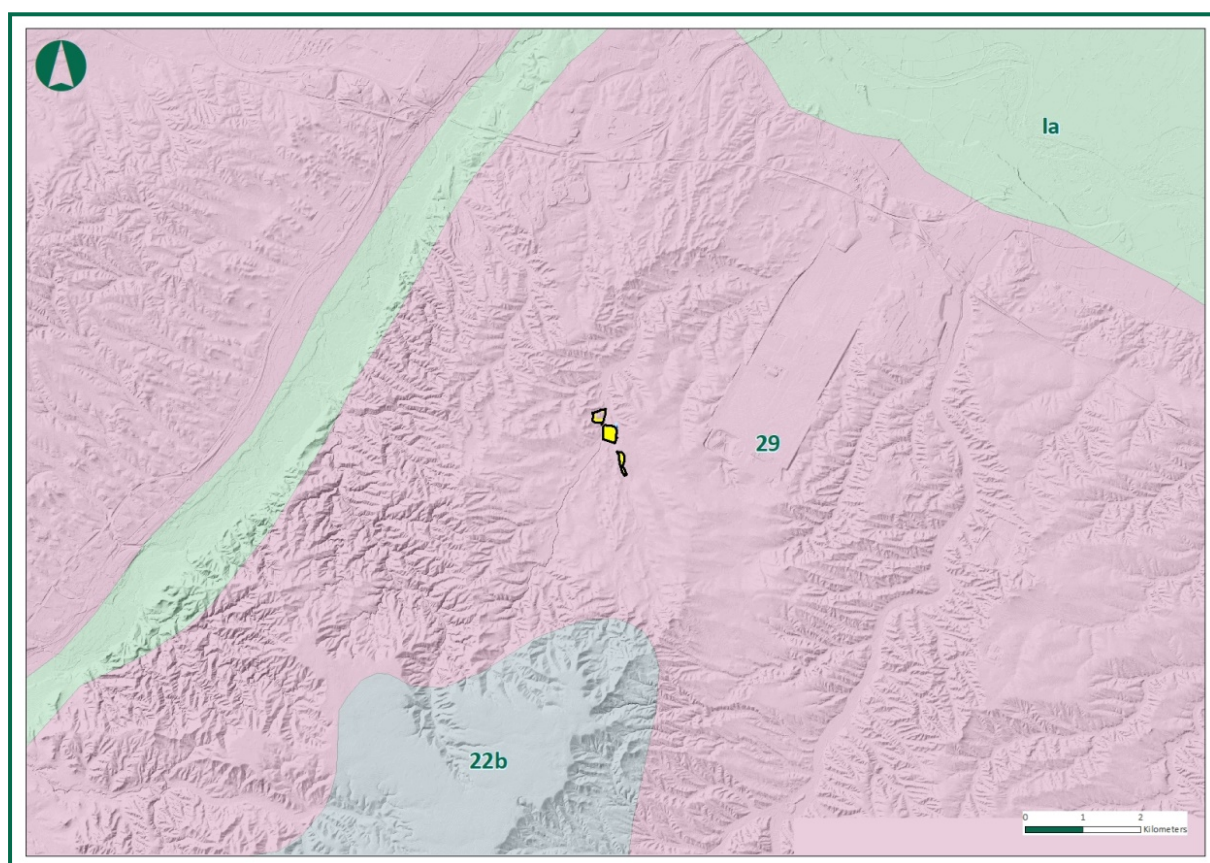
Figura 27: Vegetación potencial de la zona de estudio.
