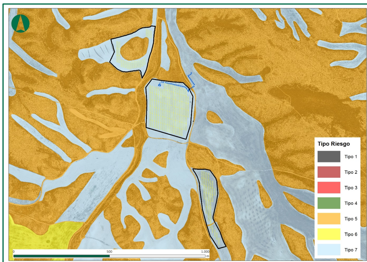
Figura 31. Zonas de riesgo de incendio forestal. Fuente: IDEARAGON.
