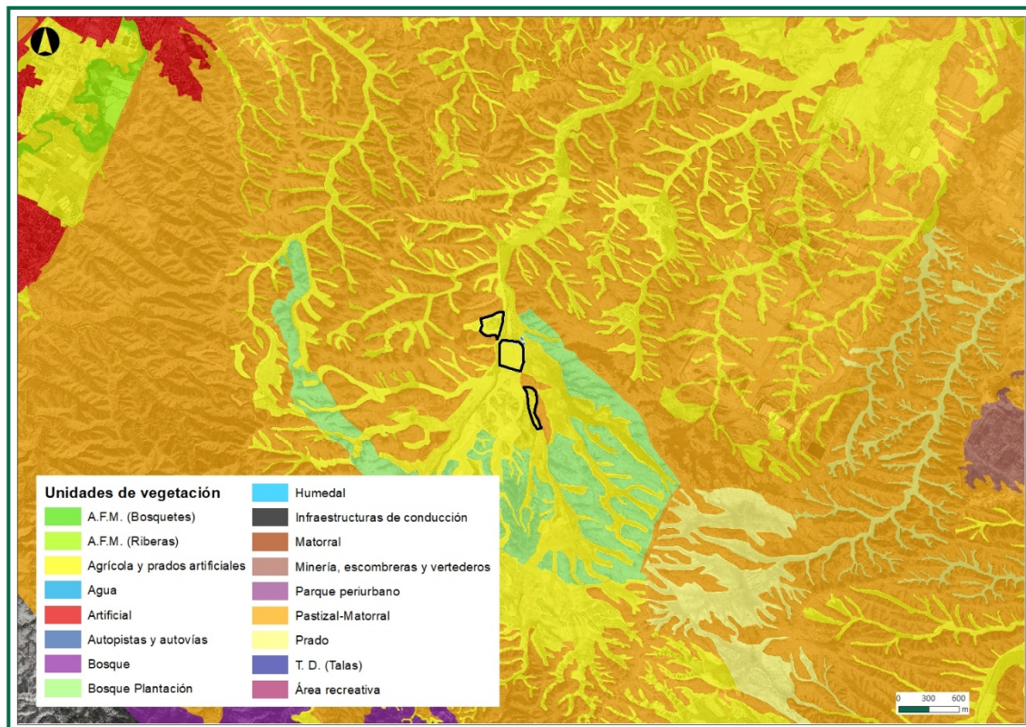
Figura 28: Unidades de vegetación
