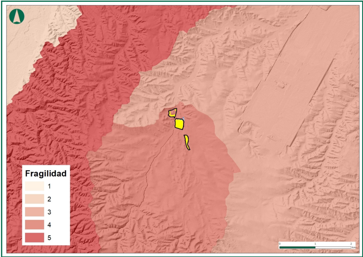
Figura 37. Índice de Fragilidad del paisaje de Comarca DC Zaragoza. Fuente: Gobierno de Aragón
