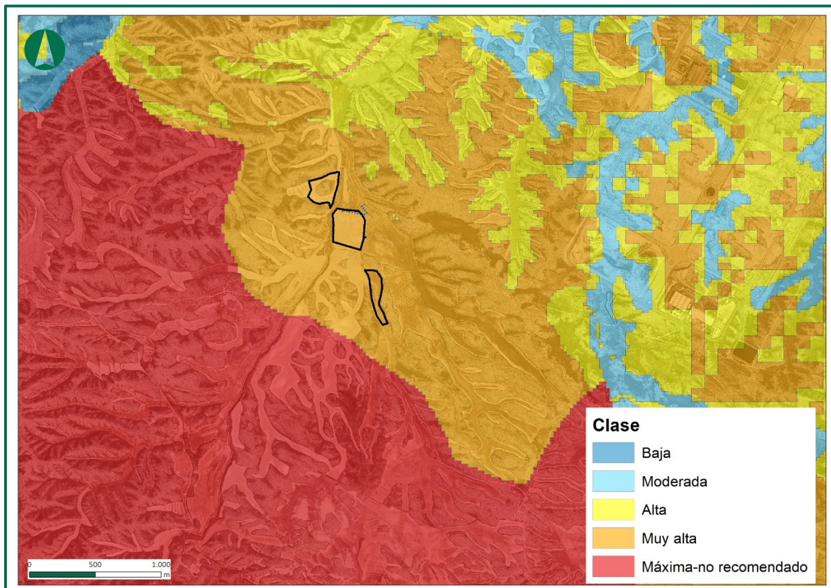
Figura 51. Zonificación de sensibilidad ambiental para energías renovables. Fuente: MITERD.
