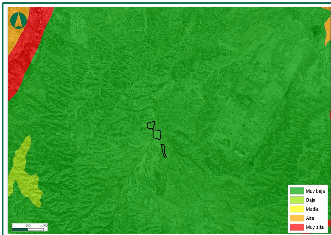
Figura 26. Permeabilidad existente en la zona de estudio. Fuente: CHE
