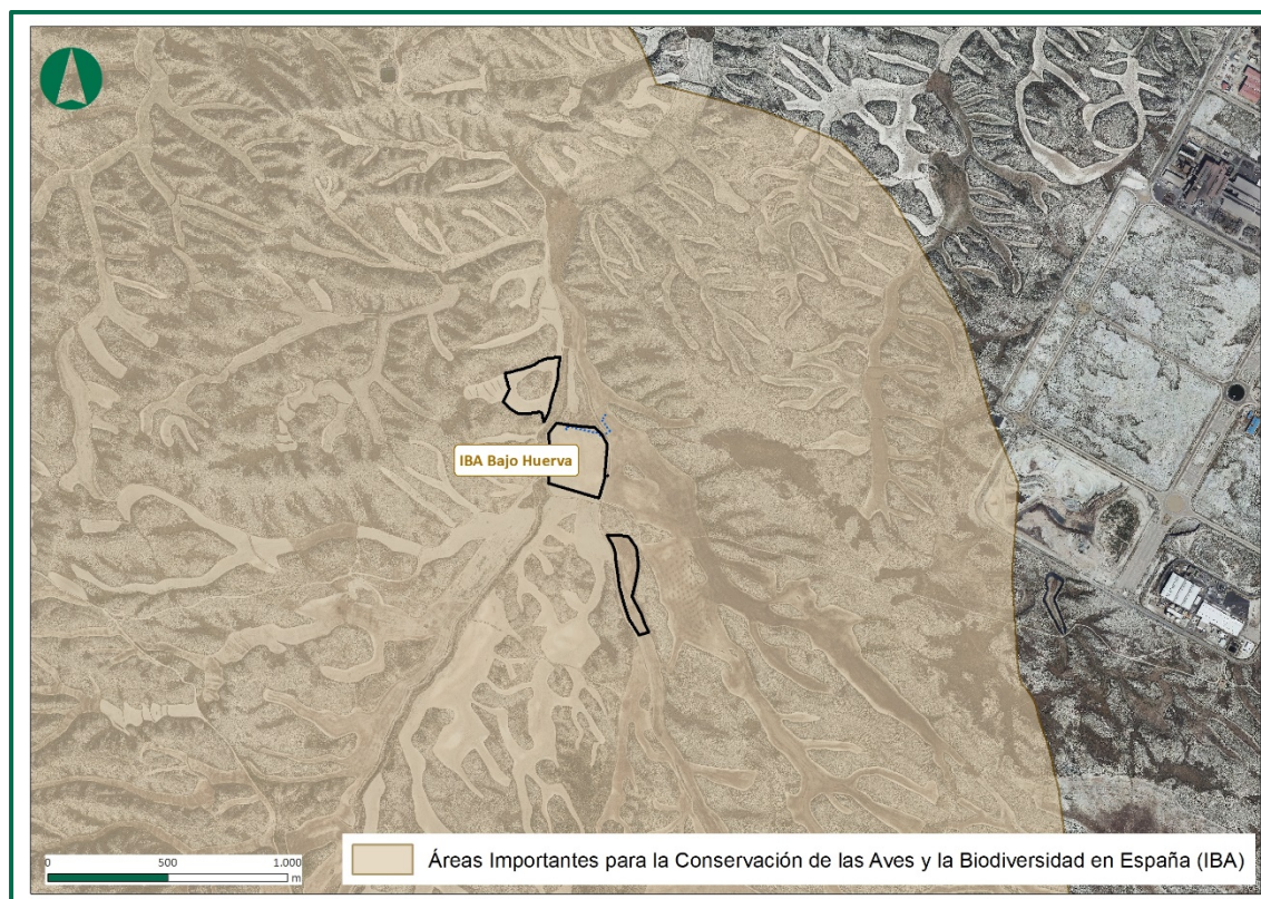
Figura 47. IBA en el entorno del área estudiada. Fuente: MITECO
