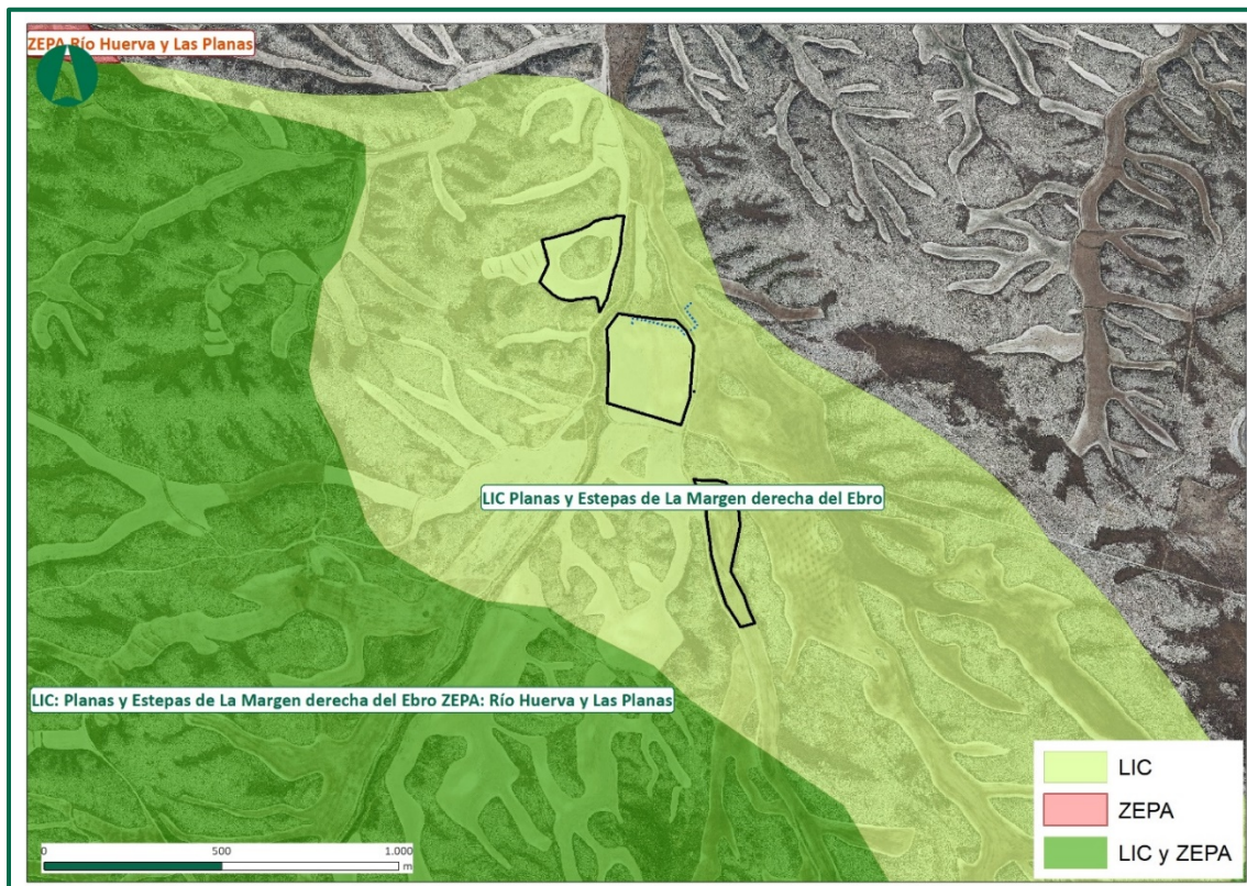
Figura 45. Red Natura 2000 en el entorno del área estudiada. Fuente: MITERD
