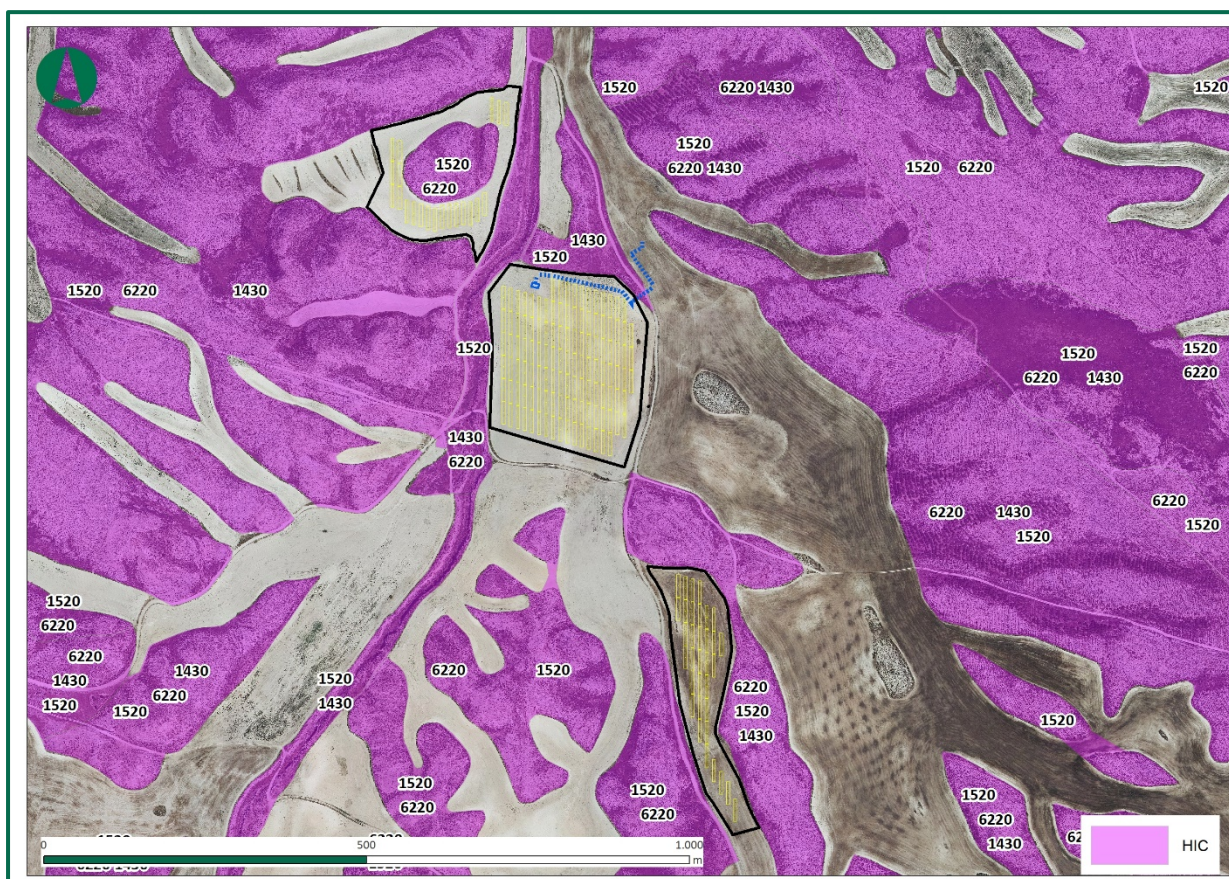
Figura 46: Hábitats Interés comunitario.
