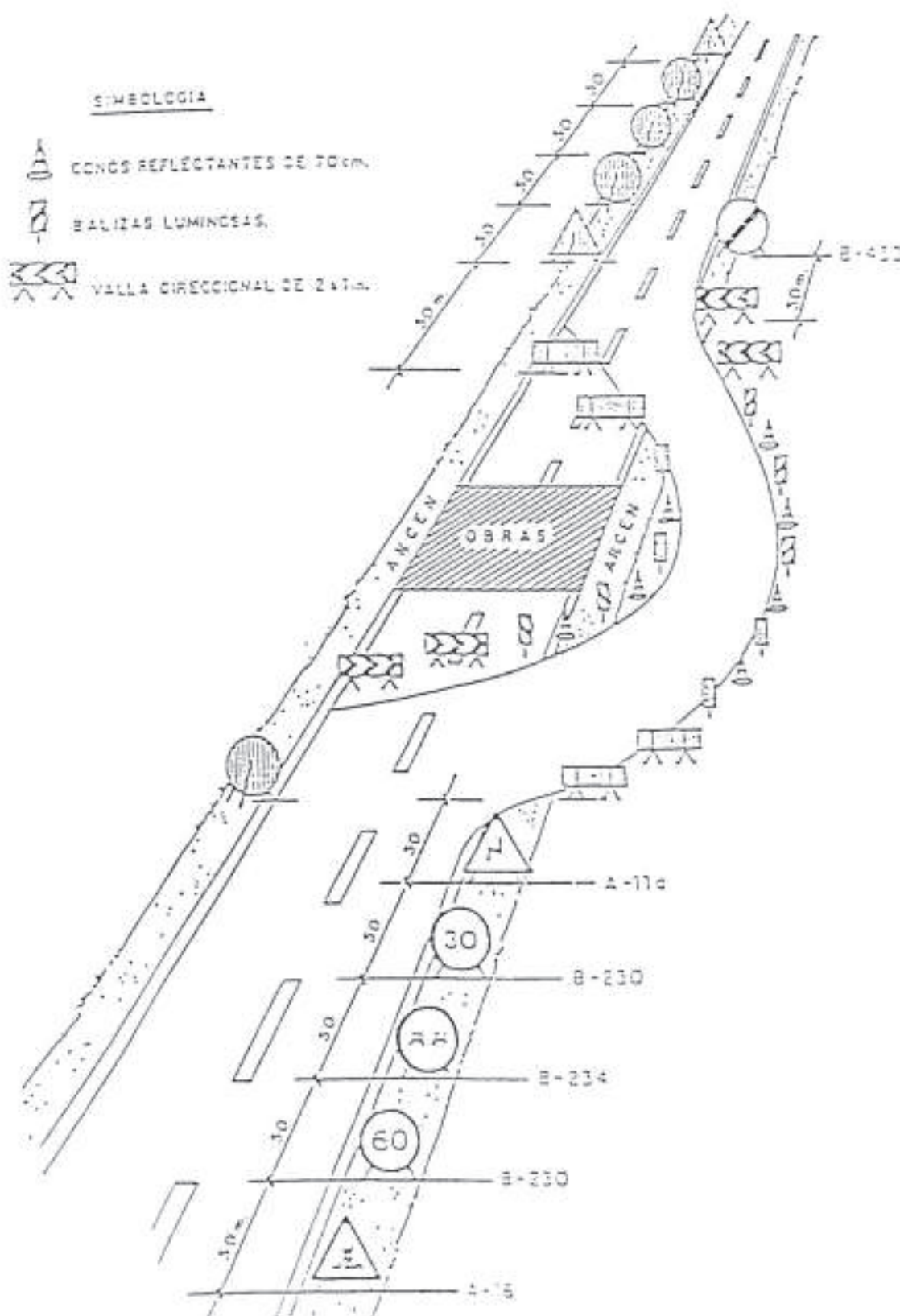
BALIZAMIENTO EN CORTES DE CARRETERA CON DESVÍO
