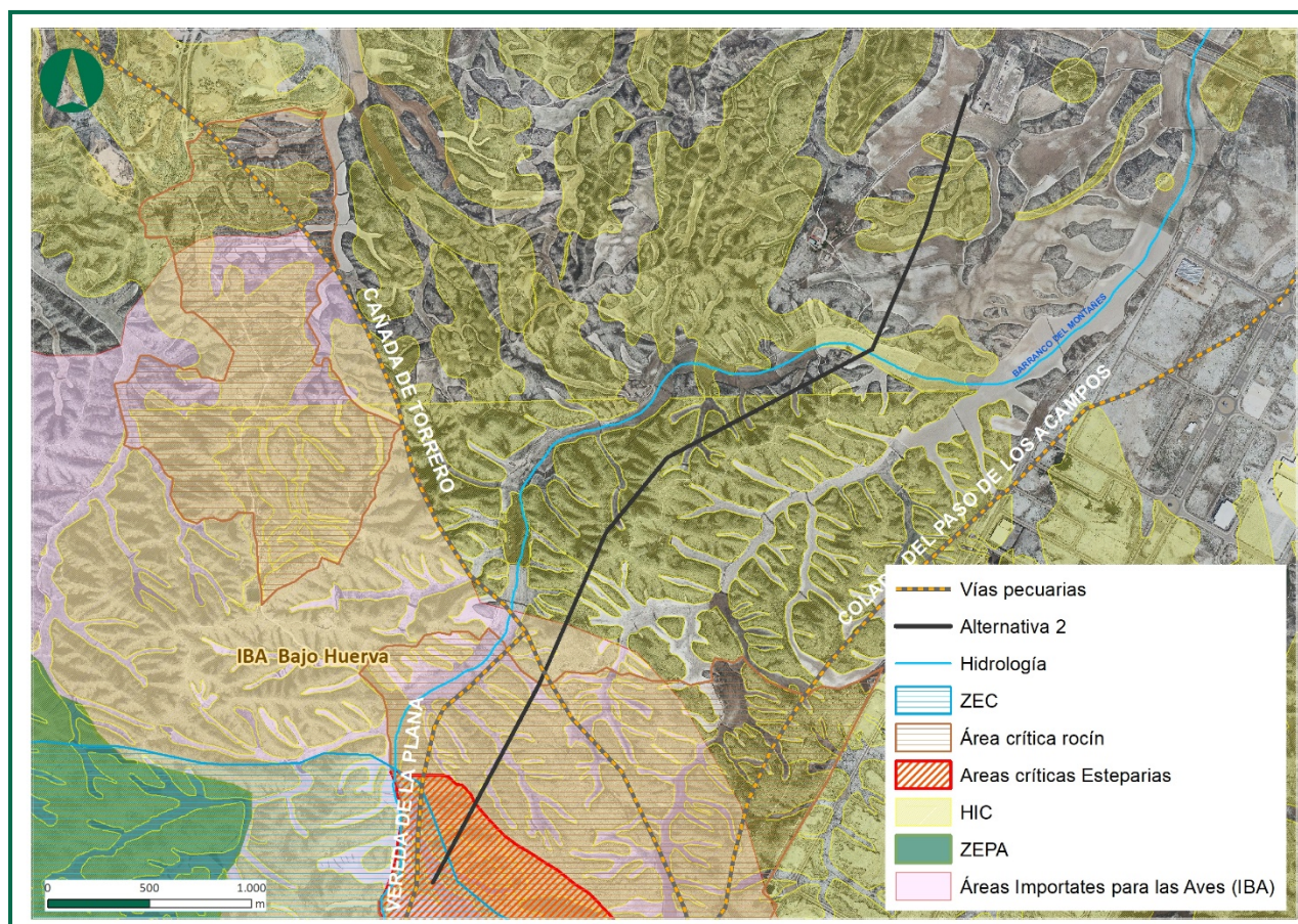
Figura 3. Alternativa 2 de LAAT
