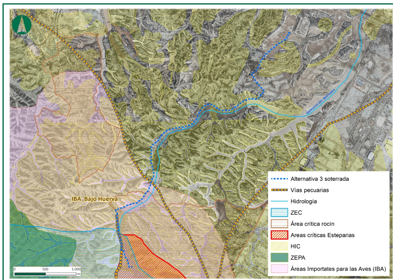
Figura 4. Alternativa 3 de línea soterrada
