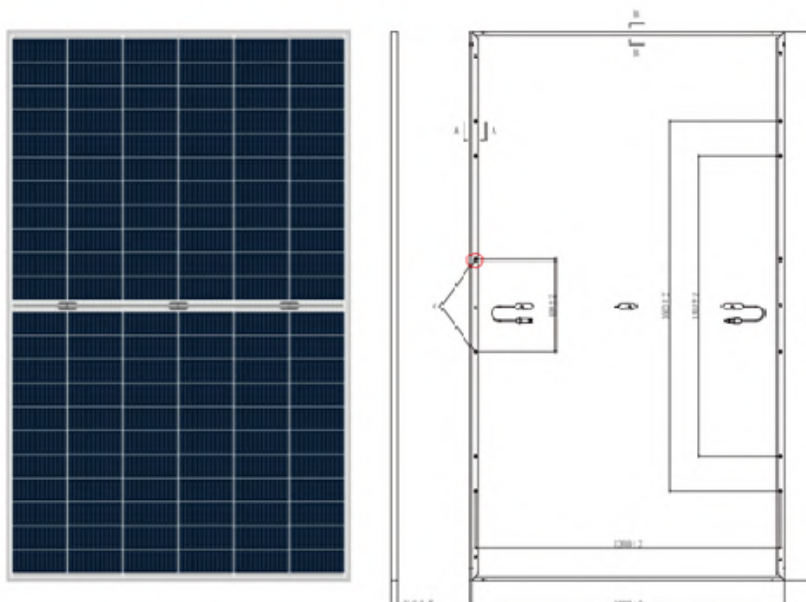
Figura 8: Dimensiones del Módulo
