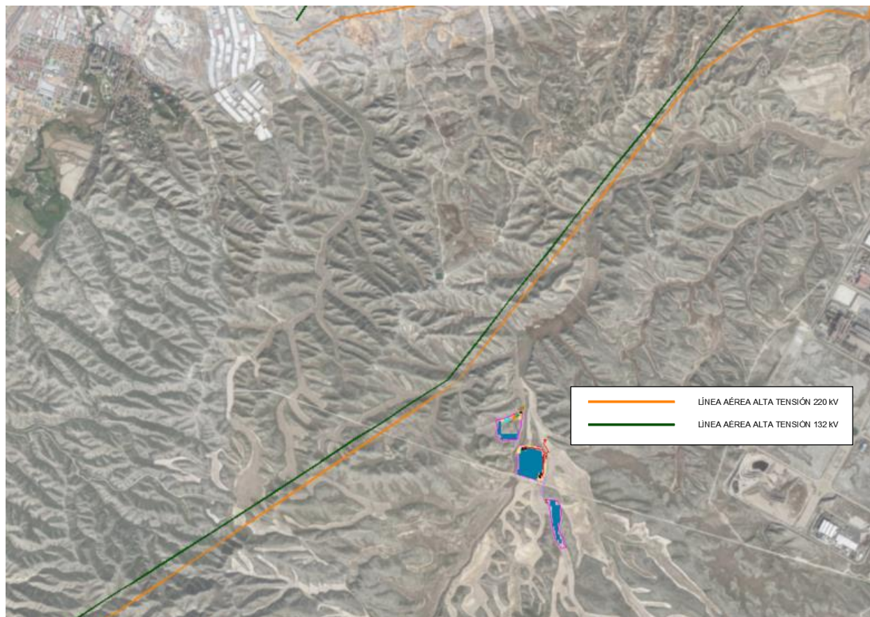
Figura 5: Líneas eléctricas.
