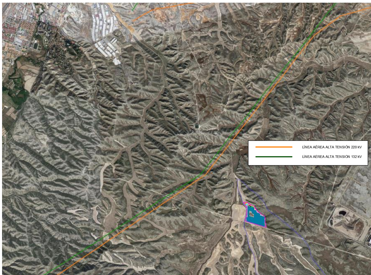
Figura 5: Líneas eléctricas.
