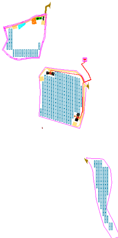
Figura 7: Lay-out de la Planta Solar
