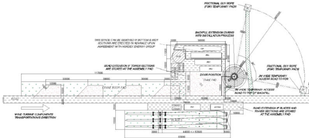
Ilustración 5. Esquema plataforma para TS118-03.
