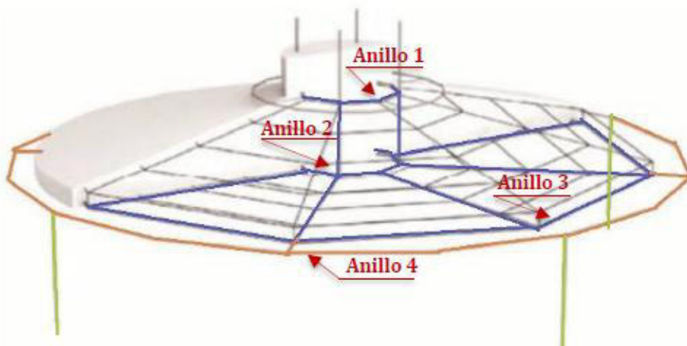
Ilustración 8. Propuesta de configuración de puesta a tierra de los aerogeneradores
