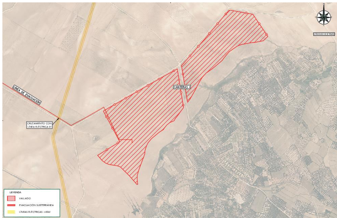
Ilustración 14 Vista afección a líneas eléctricas
