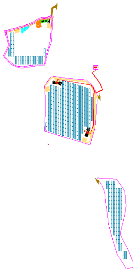
Figura 7: Lay-out de la Planta Solar
