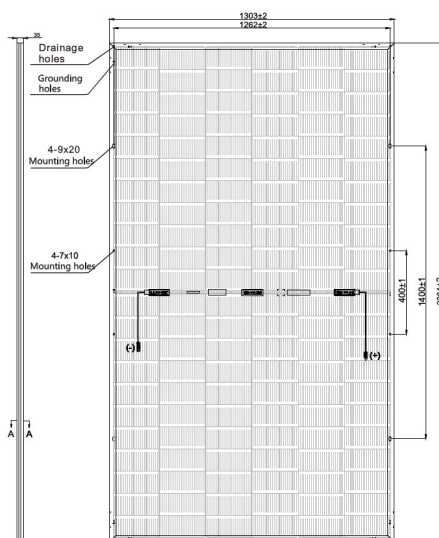
Ilustración 5. Módulo fotovoltaico
