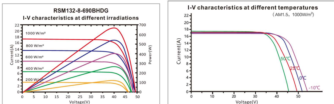
Ilustración 6. Curvas características
