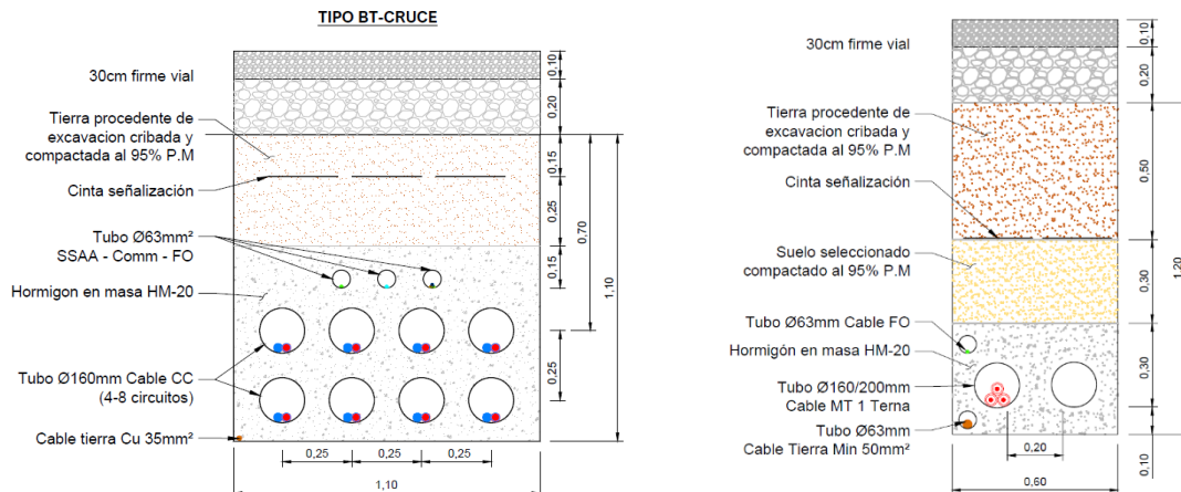
Ilustración 8: Detalles de las zanjas tipo cruce para BT (izda.) y MT (dcha.)
