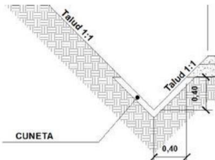
Imagen 15: Cuneta tipo
