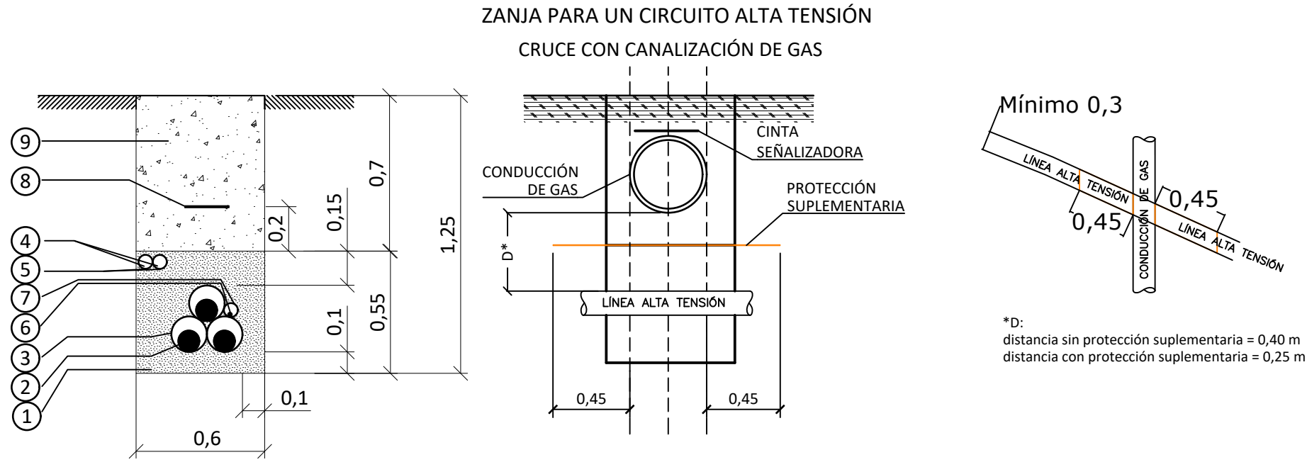
DETALLE ZANJA CRUZAMIENTO (ESCALA A1:25)
