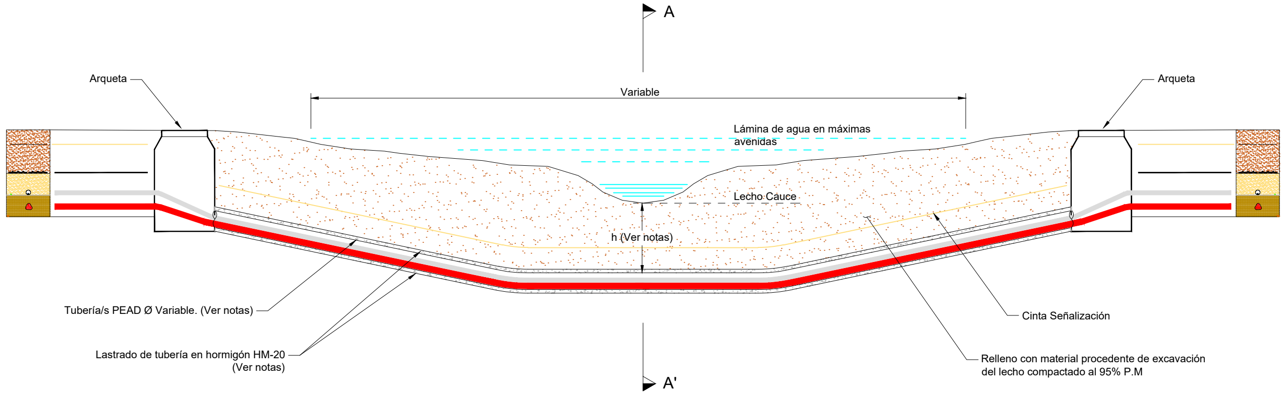
CRUZAMIENTO TIPO - ZANJA CON CAUCE
