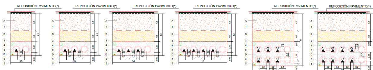
Imagen 19: zanjas tipo conductor entubado bajo viales/caminos o drenajes.
