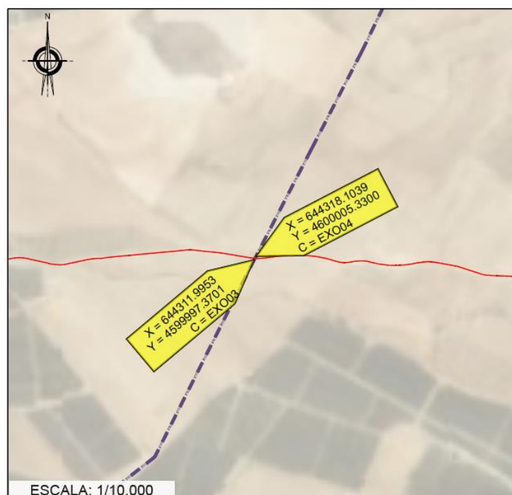
Imagen 22: Cruce de RMT con oleoducto de EXOLUM
