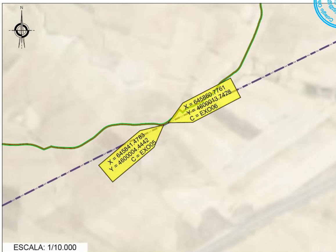
Imagen 22: paralelismo RMT con oleoducto de EXOLUM
