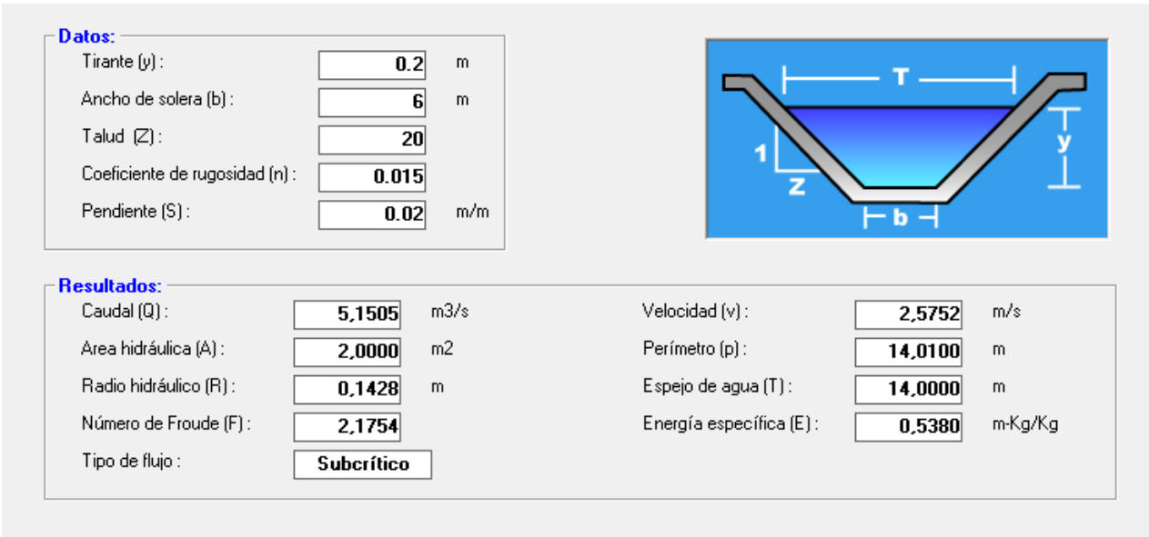
Imagen 12: Máximo caudal para vado tipo 2
