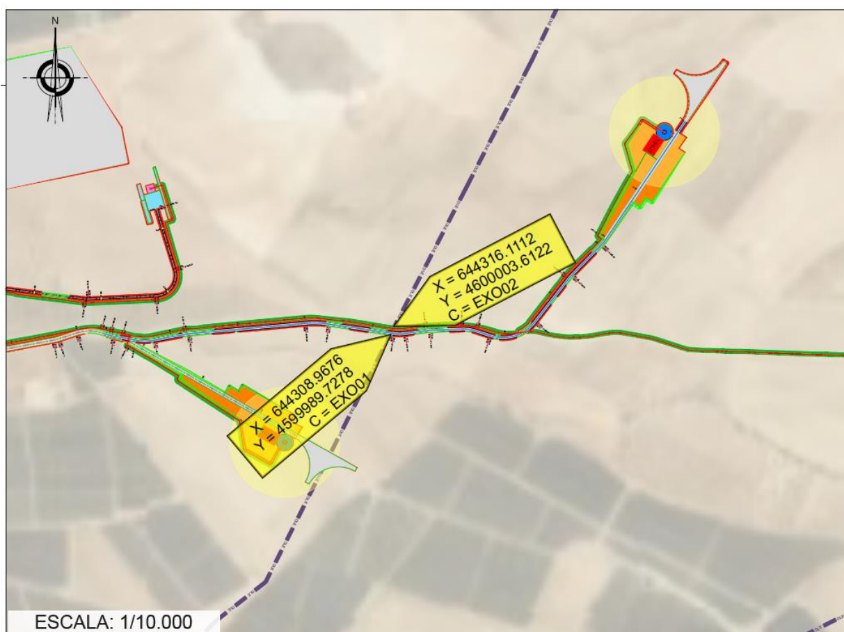
Imagen 20: cruzamiento vial y RMT con oleoducto de EXOLUM
