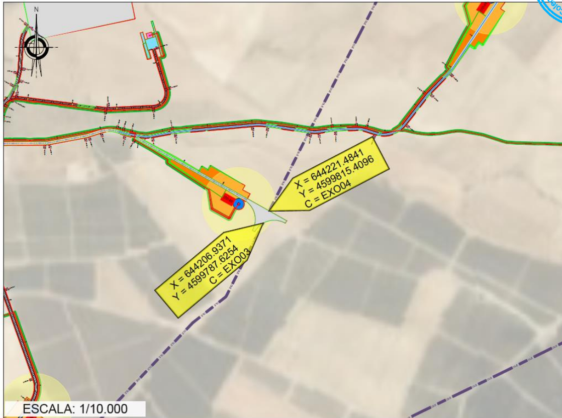
Imagen 21: Cruce zona de giro del aerogenerador LTO-02 con oleoducto de EXOLUM
