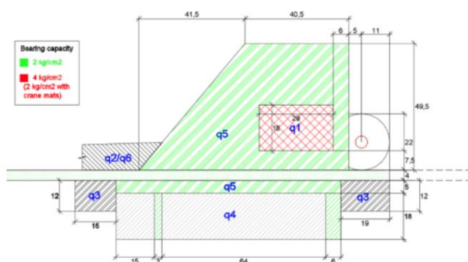
Imagen 15: Plataforma Aerogenerador N163-6.X
