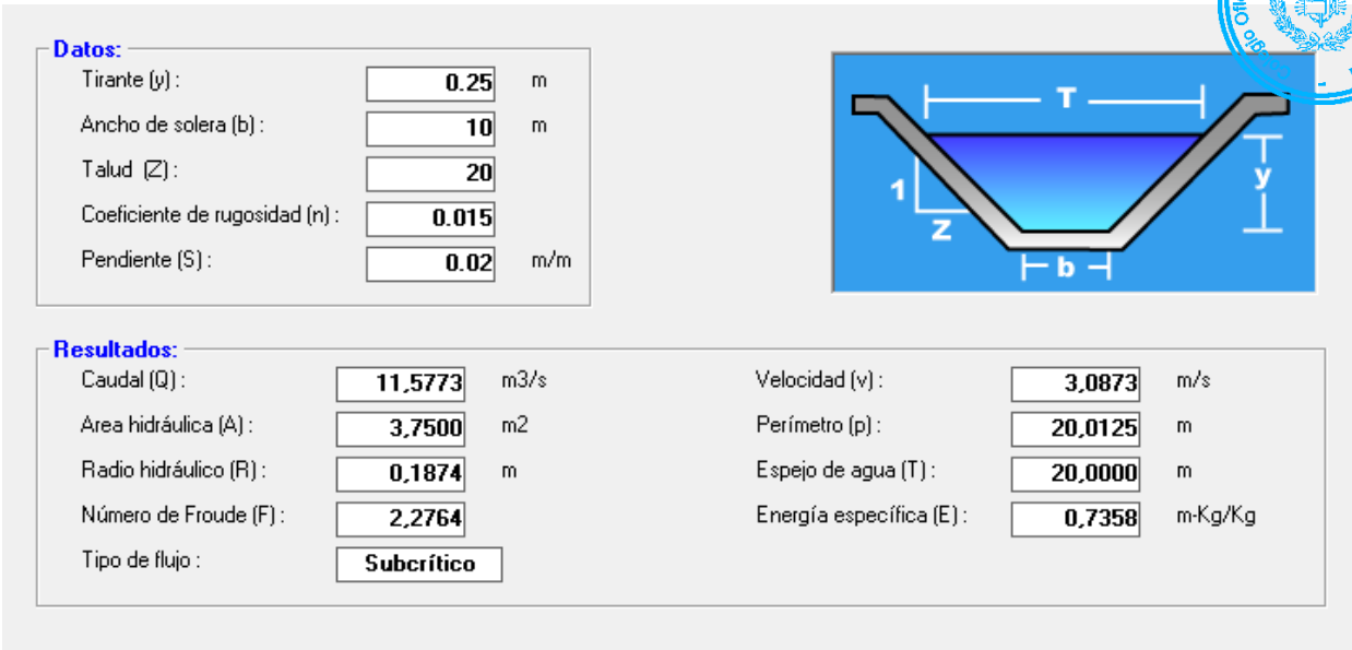
Imagen 11: Máximo caudal para vado tipo 1
