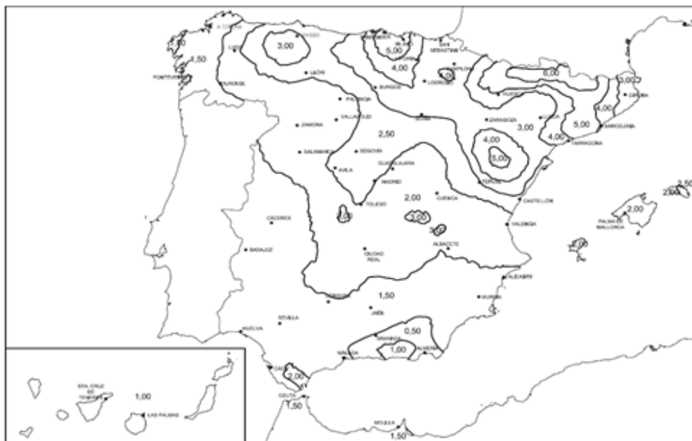
Figura 14. Mapa de densidad de impactos sobre el terreno (Figura 1.1 de la sección SUA 8 Seguridad frente al riesgo causado por la acción del rayo)
