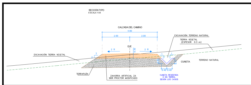
Figura 7. Sección tipo
