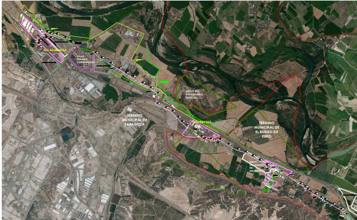
Situación de línea aero subterránea en TT.MM de Zaragoza y El Burgo de Ebro, desde SET Alumnisa, realizando entrada-salida en SET Prydes hasta entronque con línea existente Prydes-El Burgo en apoyo 99 existente.
