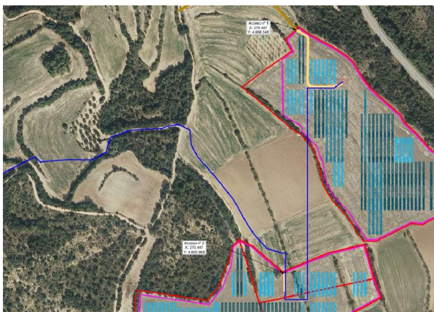
Ilustración 3. Accesos a la planta solar (1/2)
