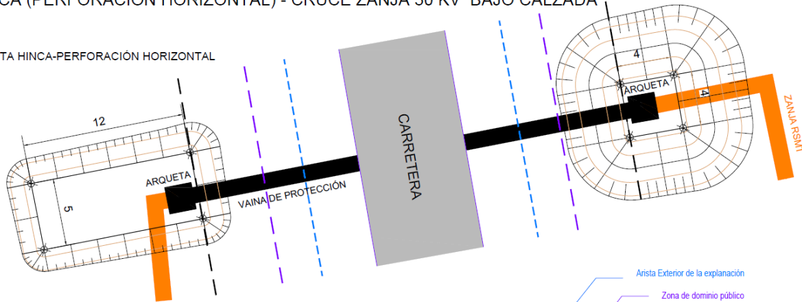
PERFIL HINCA-PERFORACIÓN HORIZONTAL
